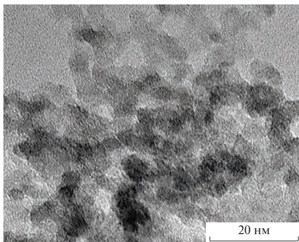
Рис. 3. Типичное ПЭМ-изображение нанодисперсных частиц оксида меди (образец РГ5).
