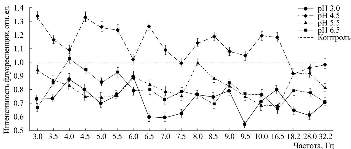
Рис. 4. Усредненные зависимости интегральной интенсивности флуоресценции растворов ЧСА ( 1 \cdot 10^{-6} М) от частоты ЭМП при разных значениях pH. Время обработки образцов 15 мин, t = 23^\circ\text{C} .
