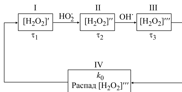
Рис. 5. Схема взаимопревращений перекиси водорода в водном растворе биополимера в ходе протекания реакций (1)–(10).
