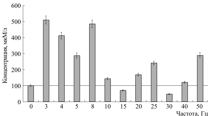
Рис. 2. Содержание перекиси водорода до (0 Гц) и после воздействия ЭМП с различными частотами в водных растворах ДНК с концентрацией 0.025 мкг/мл, время обработки образцов 30 мин, t = 21^\circ\text{C} .
