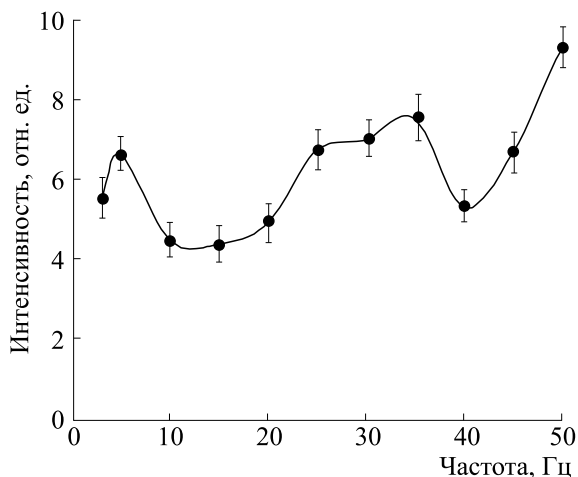
Рис. 1. Усредненная зависимость интенсивности флуоресценции при \lambda_{\text{max}} = 645 \pm 5 нм растворов ДНК с концентрацией 0.025 мкг/мл от частоты ЭМП. Время обработки образцов 30 мин, t = 21^\circ\text{C} .
