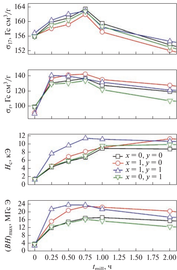
Рис. 3. Зависимости гистерезисных свойств порошка \text{Sm}_2\text{Fe}_{17}\text{N}_3 , измельченного в среде ацетона без добавок ( x = 0, y = 0 ), с добавкой 1% МК ( x = 1, y = 0 ), 1% СО ( x = 0, y = 1 ) и 1% МК + 1% СО ( x = 1, y = 1 ) от t_{\text{mill}} .
