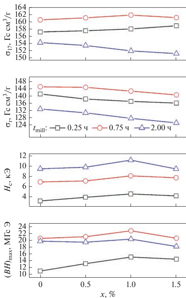
Рис. 2. Зависимость гистерезисных свойств порошка \text{Sm}_2\text{Fe}_{17}\text{N}_3 от концентрации метилкапроата ( x ) при времени помола t_{\text{mill}} = 0.25; 0.75 и 2 ч.
