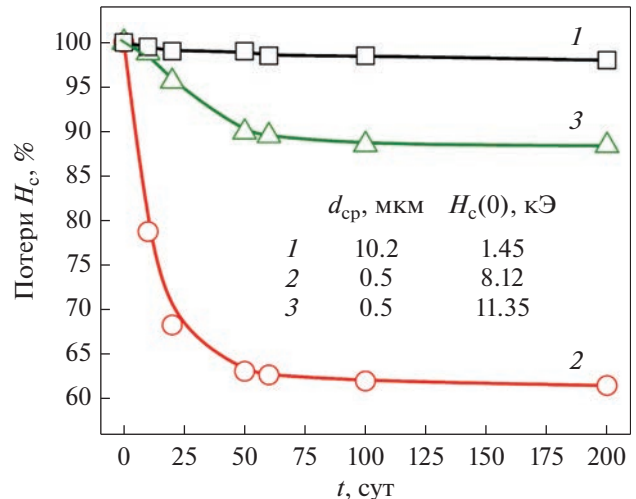
Рис. 7. Зависимости снижения H_c порошков Sm_2Fe_{17}N_3 от времени хранения на воздухе: (1) исходный крупнозернистый порошок; (2) порошок, измельченный с добавкой 1% МК; (3) порошок, измельченный с добавкой и 1% МК и 1% СО.
