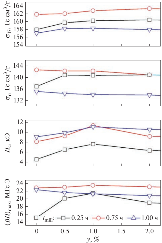
Рис. 4. Зависимость гистерезисных свойств порошка \text{Sm}_2\text{Fe}_{17}\text{N}_3 от концентрации силоксана ( y ), добавляемого в защитную жидкость (ацетон + 1% МК), при времени помола t_{\text{mill}} = 0.25; 0.75 и 1 ч.
