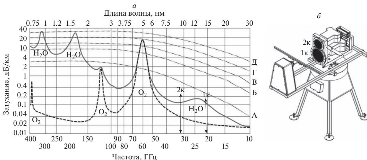
Рис. 1. (а) — величина поглощения сигнала в земной атмосфере в миллиметровом диапазоне волн. Сплошная кривая — затухание для стандартной модели атмосферы (учтены главные газовые составляющие — \text{H}_2\text{O} и \text{O}_2 ). Штриховая кривая — затухание в “сухой атмосфере” (без паров воды). Пунктирные кривые А–Д — поглощение в жидкой фазе воды (в дожде): А — 0.25 мм/ч (слабый дождь), Б — 12.5 мм/ч (умеренный дождь), В — 25 мм/ч (сильный дождь), Г — 50 мм/ч (ливень), Д — 100 мм/ч (тропический ливень). Двойными стрелками (1к, 2к) отмечены положения рабочих частот РВП. (б) — схема расположения блоков СВЧ-приемников РВП с коническими РЛА. 1к — канал А (20.7 ГГц), 2к — канал Б (31.4 ГГц).
