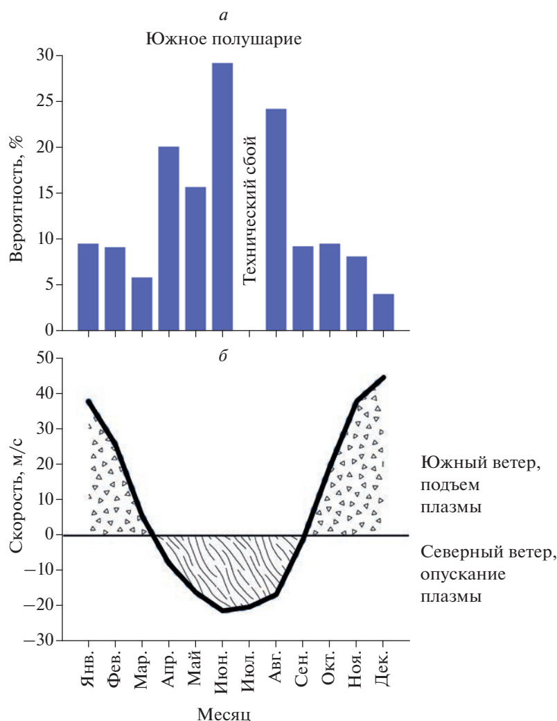
Рис. 1. (а) Вариации P_{EPB} , построенные в зависимости от месяца года для Южного полушария. Ежемесячные значения P_{EPB} являются медианами по среднеширотному интервалу наблюдений (25^{\circ}-55^{\circ}) DIPLAT. Данные спутника ISS-b ( \sim 972-1220 км) за полтора года наблюдений (август 1978–декабрь 1979 гг.). (б) Месячные модельные вариации скорости меридионального термосферного ветра, рассчитанные над экватором на высоте \sim 400 км (черная сплошная кривая). Расчет по модели горизонтальных ветров HWM14 [Drob et al., 2015]. Положительные значения скорости соответствуют южным ветрам, отрицательные – северным. Области, заполненные треугольниками и штриховыми линиями, соответствуют областям подъема и опускания плазмы в Южном полушарии.
