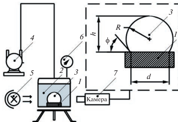
Рис. 1. Схема экспериментальной установки для наблюдения за изменениями контактного угла сидящего пузырька. 1, исследуемые пластины 2, герметичная кювета, заполненная водой 3, воздушный пузырек 4, насос для создания вакуума 5, осветитель 6, вакуумметр 7, видеокамера.
