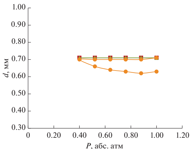
Рис. 9. Зависимость диаметра посадочной d сидящего пузырька от давления (для 4-х циклов). Прямые зависимости сливаются в одну линию.
