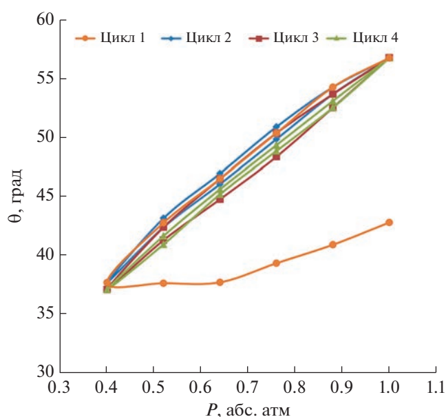
Рис. 7. Зависимость значений контактных углов сидящего пузырька на поверхности слюды с начальным углом смачивания 43^\circ от внешнего давления. Четыре цикла измерений.
