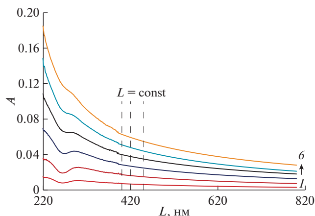
Рис. 2. Спектры A(\lambda) для наномэмульсий Бридж L4 с различными его концентрациями (через 14 дней): 1 – 0.063; 2 – 0.124; 3 – 0.184; 4 – 0.243; 5 – 0.300 и 6 – 0.356 мМ.
