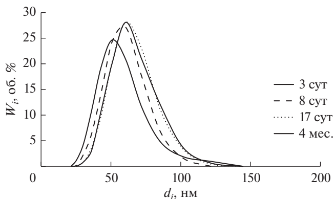
Рис. 5. Дифференциальные кривые распределения частиц по размерам наноэмульсии Бридж L4 ( C_{\text{Бр-4}} = 84.1 мМ) при различных временах хранения (время указано в легенде).
