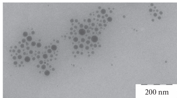
Рис. 11. Микрофотография наноэмульсии Бридж L4 ( C_{\text{Бр-4}} = 166.8 \text{ mM} ) с ХГ, полученная методом ПЭМ через 1 мес. хранения.
