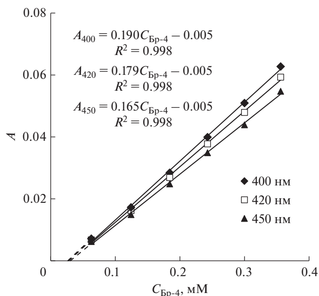
Рис. 3. Зависимости оптической плотности предельно разбавленных прямых наномэмульсий Бридж L4 от его концентрации при длинах волн 400, 420 и 450 нм.
