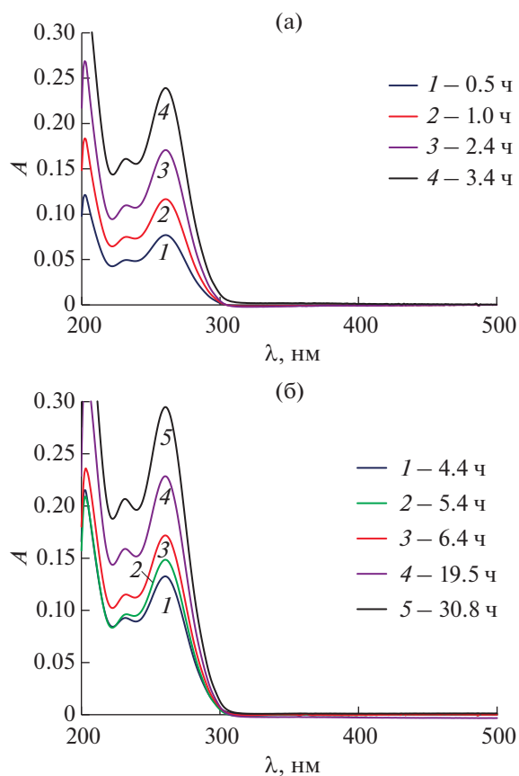
Рис. 12. Спектры поглощения проб приемной среды из ячейки Франца при различных временах наблюдения (время указано в легенде) для определения массопереноса ХГ частицами дисперсной фазы наноэмульсий Бридж L4 ( C_{Бр-4} = 166.8 мМ). Пробы разбавлены n -пропиловым спиртом (а – в 16.7 раз; б – в 34.3 раза). Раствор сравнения – приемная среда, разбавленная n -пропиловым спиртом в такое же количество раз.
