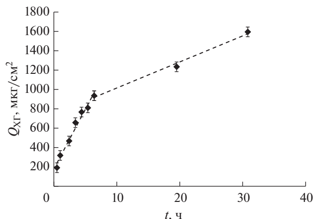
Рис. 13. Кинетика массопереноса ХГ частицами дисперсной фазы наноэмульсий Бридж L4 ( C_{\text{Бр-4}} = 166.8 \text{ мМ} ).
