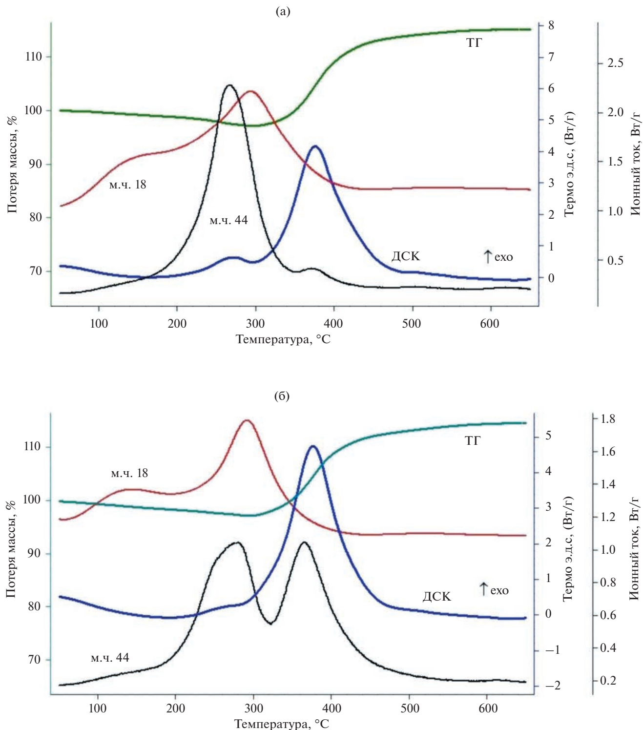
Рис. 5. Комплексные термограммы нагрева МНЧ Ni/G06 (а) и Ni@C/G06 (б) с регистрацией изменения массы образца (ТГ), тепловыделения (б) и выделения летучих продуктов с массовыми числами (м.ч.) 18 и 44.
