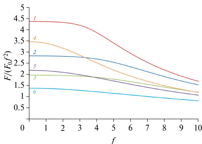
Рис. 5. Зависимость нормированной силы электростатического взаимодействия частиц от f при h/a = 0.1 : 1 – k = 0.1 , \varepsilon = 0.1 ; 2 – k = 0.1 , \varepsilon = 1 ; 3 – k = 0.1 , \varepsilon = 10 ; 4 – k = 1 , \varepsilon = 0.1 ; 5 – k = 1 , \varepsilon = 1 ; 6 – k = 1 , \varepsilon = 10 .
