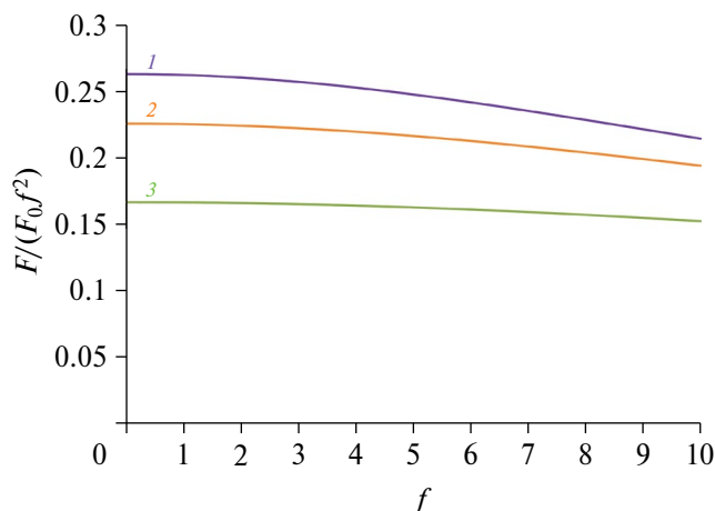
Рис. 6. Зависимость нормированной силы электростатического взаимодействия частиц от f при h/a = 0.1 и k = 10 : 1 – \varepsilon = 0.1 ; 2 – \varepsilon = 1 ; 3 – \varepsilon = 10 .
