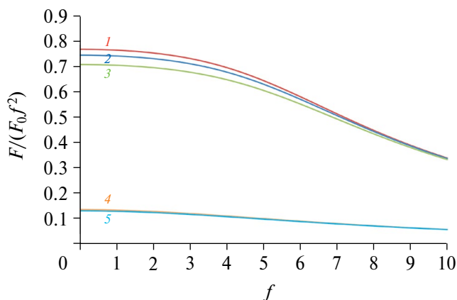
Рис. 7. Зависимость нормированной силы электростатического взаимодействия частиц от f при h/a = 2 : 1 – k = 0.1 , \varepsilon = 0.1 ; 2 – k = 0.1 , \varepsilon = 1 ; 3 – k = 0.1 , \varepsilon = 10 ; 4 – k = 1 , \varepsilon = 0.1 ; 5 – k = 1 , \varepsilon = 10 .
