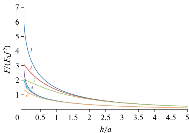
Рис. 2. Зависимость нормированной силы электростатического взаимодействия частиц от нормированного расстояния между поверхностями частиц при k = 1 : 1 – f = 1 , \varepsilon = 0.1 ; 2 – f = 1 , \varepsilon = 1 ; 3 – f = 1 , \varepsilon = 10 ; 4 – f = 10 , \varepsilon = 0.1 ; 5 – f = 10 , \varepsilon = 1 ; 6 – f = 10 , \varepsilon = 10 .
