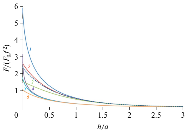
Рис. 3. Зависимость нормированной силы электростатического взаимодействия частиц от нормированного расстояния между поверхностями частиц при k = 10 : 1 – f = 1 , \varepsilon = 0.1 ; 2 – f = 1 , \varepsilon = 1 ; 3 – f = 1 , \varepsilon = 10 ; 4 – f = 10 , \varepsilon = 0.1 ; 5 – f = 10 , \varepsilon = 1 ; 6 – f = 10 , \varepsilon = 10 ; пунктирная линия – LS приближение.
