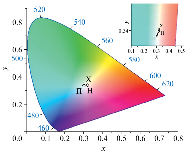
Рис. 7. Смещение цветового тона ОСП на основе кремнийорганического лака КО-921, модифицированных 17 масс. % ПДМС и 20 масс. % эпоксидной смолы. На врезке: смещение цветового тона \Delta E в условиях тропического саванного (Нячанг — Н) и субэкваториального климата (Хошимин — Х) за 16 месяцев экспозиции по отношению к моменту постановки (П).
