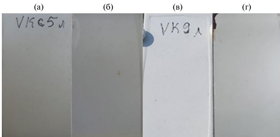
Рис. 8. Фотоснимки, иллюстрирующие изменение состояния поверхности ОСП на основе кремнийорганического лака КО-921, модифицированных 17 масс. % ПДМС и 20 масс. % эпоксидной смолы, за время экспозиции в Троп-центре (СР Вьетнам): а) исходное состояние при постанове на МНИИС Дам Бай, б) через 16 месяцев в тропическом саванном климате; в) исходное состояние при постанове на КИС Кон Зо; г) спустя 16 месяцев в субэкваториальном климате.
