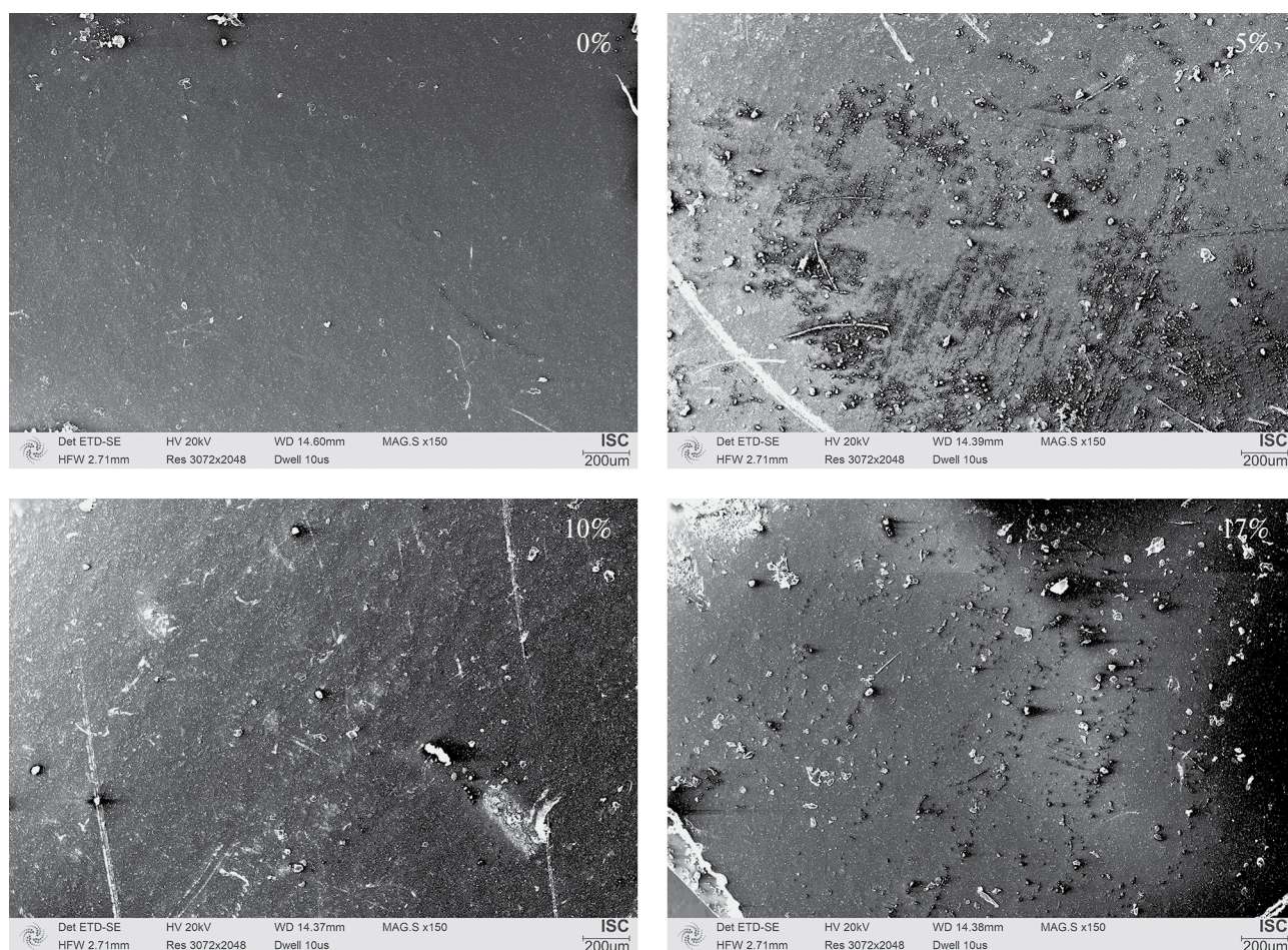
Рис. 3. СЭМ-изображения покрытий на основе кремнийорганического лака КО-921 с разной концентрацией ПДМС.
