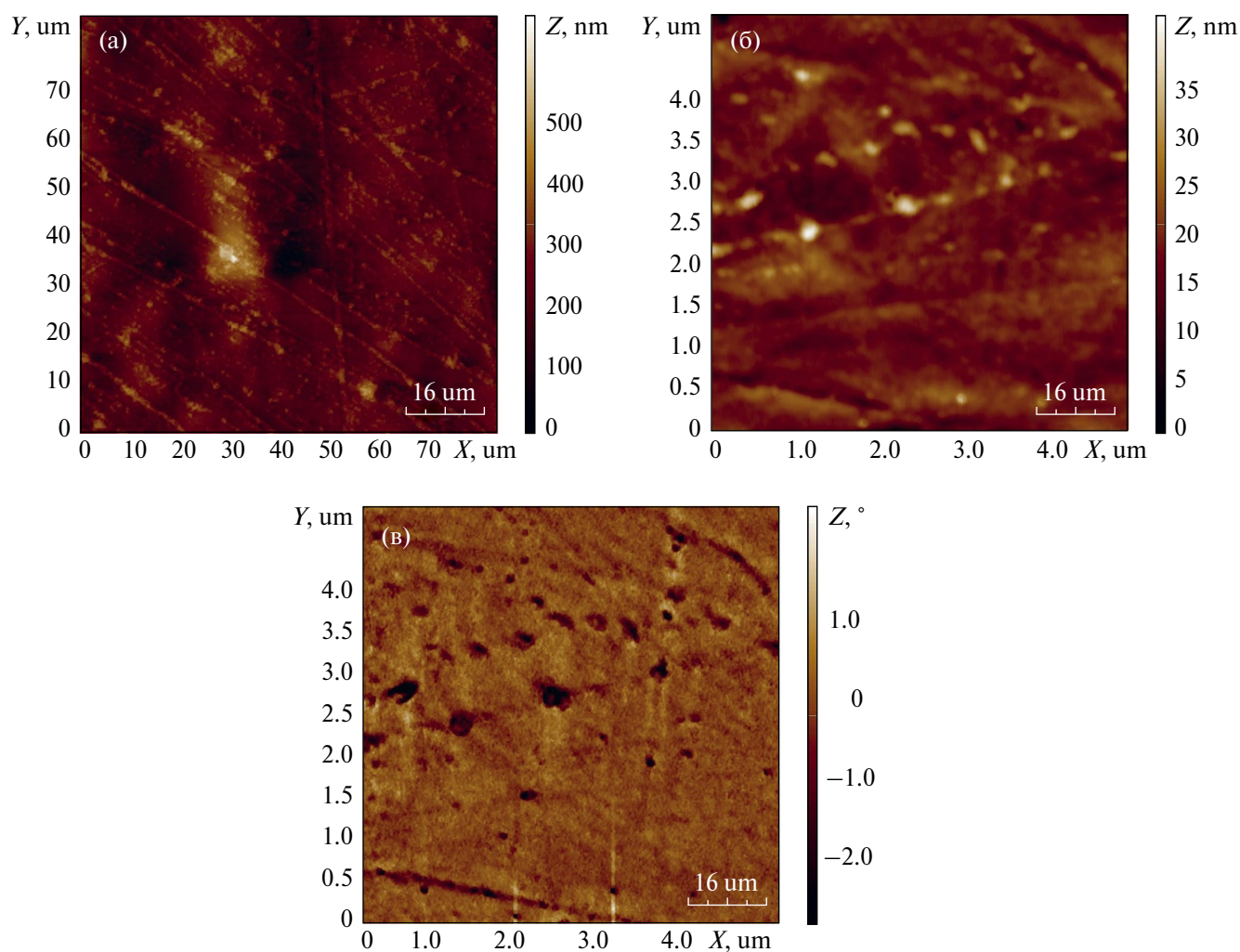
Рис. 2. АСМ-изображения покрытий из ОСК на основе лака КО-921, без ПДМС. а, б) топология; в) фазовый контраст.
