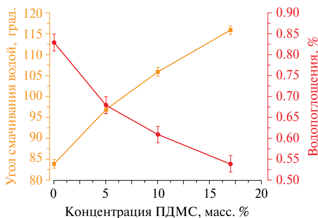
Рис. 4. Зависимости степени гидрофобности и водопоглощения ОСП на основе кремнийорганического лака КО-921, от концентрации модифицирующей добавки ПДМС: • – угол смачивания водой, ■ – водопоглощение.
