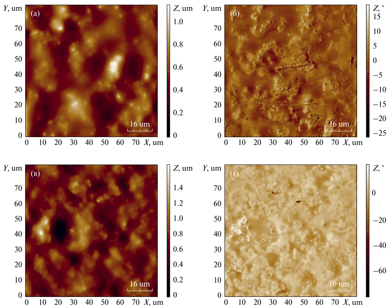
Рис. 1. АСМ-изображения покрытий из ОСК на основе кремнийорганического лака КО-921, модифицированных 17 масс. % ПДМС с отвердителями: а, б) – 0/2 масс. % ТБТ; в, г) – 2 масс. % АГМ-9.
