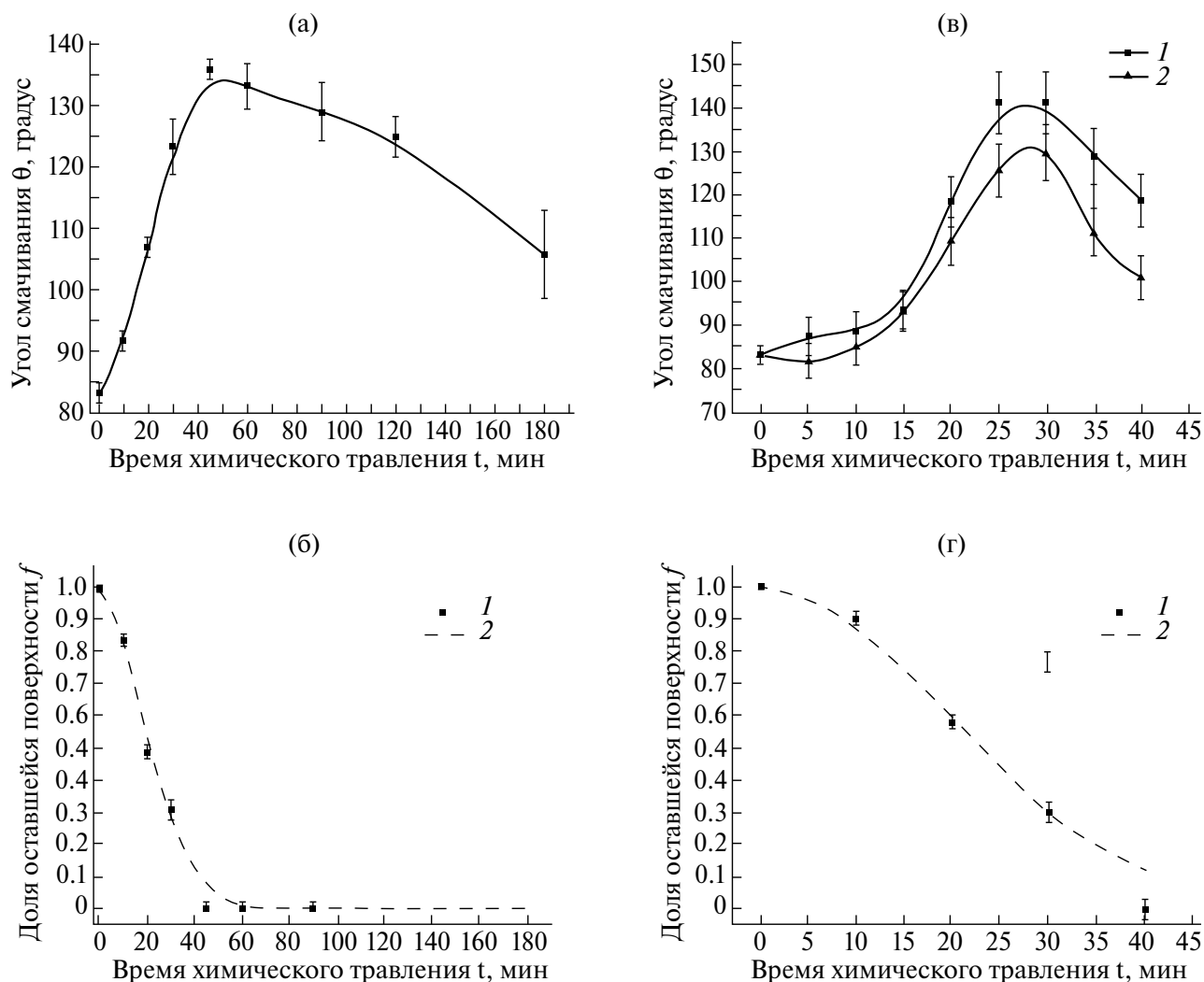
Рис. 5. Характеристики рельефов, полученных при травлении поликарбоната, облученного под углом 90° (а, б) и 45° (в, г). а, в) зависимости краевых углов от времени травления (гладкие кривые проведены от руки); б, г) зависимости доли оставшейся поверхности от времени травления: 1 – экспериментальные данные, 2 – аппроксимирующие кривые, построенные при значениях V_B = (2.15 \pm 0.16) \times 10^{-6} (б) и (1.79 \pm 0.18) \times 10^{-6} см/мин (г). Здесь и в подписи рис. 8 указаны два стандартных отклонения для величины V_B . На графике (в) приведены значения КУ слева (1) и справа (2).
