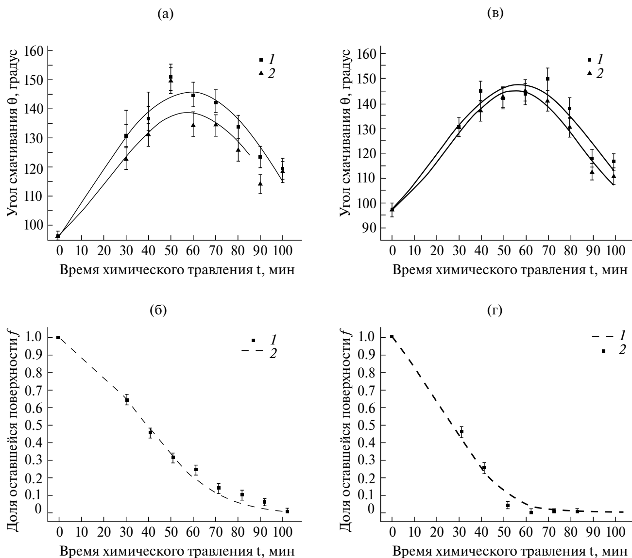
Рис. 8. Характеристики рельефов, полученных при травлении полипропилена, облученного под углом 45° (а, б) и 30° (в, г). а, в) зависимости краевых углов от времени травления. Гладкие кривые проведены от руки. На графиках приведены значения КУ слева (1) и справа (2). б, г) зависимости доли оставшейся поверхности от времени травления: 1 – экспериментальные данные, 2 – аппроксимирующие кривые, построенные при значениях V_B = (4.98 \pm 0.22) \times 10^{-6} (б) и (4.98 \pm 0.28) \times 10^{-6} см/мин (г).
