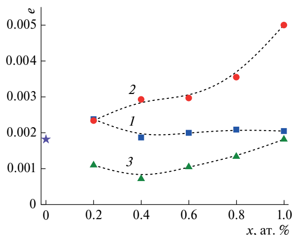
Рис. 2. Зависимость микронапряжения ( \epsilon ) от концентрации допанта ( x ) для серий покрытий x -Nb-TiO 2 (1), x -Sc-TiO 2 (2) и x -Al-TiO 2 (3). Символ “звездочка” указывает значение для покрытия недопированного диоксида титана.
