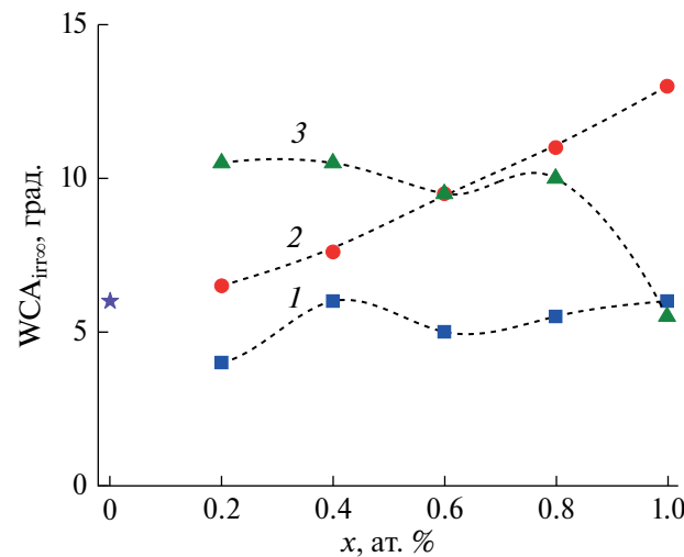
Рис. 7. Зависимости значений контактных углов воды с поверхностью, достигаемых при бесконечно долгом облучении УФ светом, ( WCA_{грд.} ) для серий покрытий x\text{-Nb-TiO}_2 (1), x\text{-Sc-TiO}_2 (2) и x\text{-Al-TiO}_2 (3) от содержания допанта. Символ “звездочка” указывает значение для недопированного диоксида титана. Плотность действующего УФ-света равна 0.5\text{ мВт/см}^2 . Значения WCA_{грд.} определены из аппроксимации кинетических данных (см. рис. П8–П10 Приложения).
