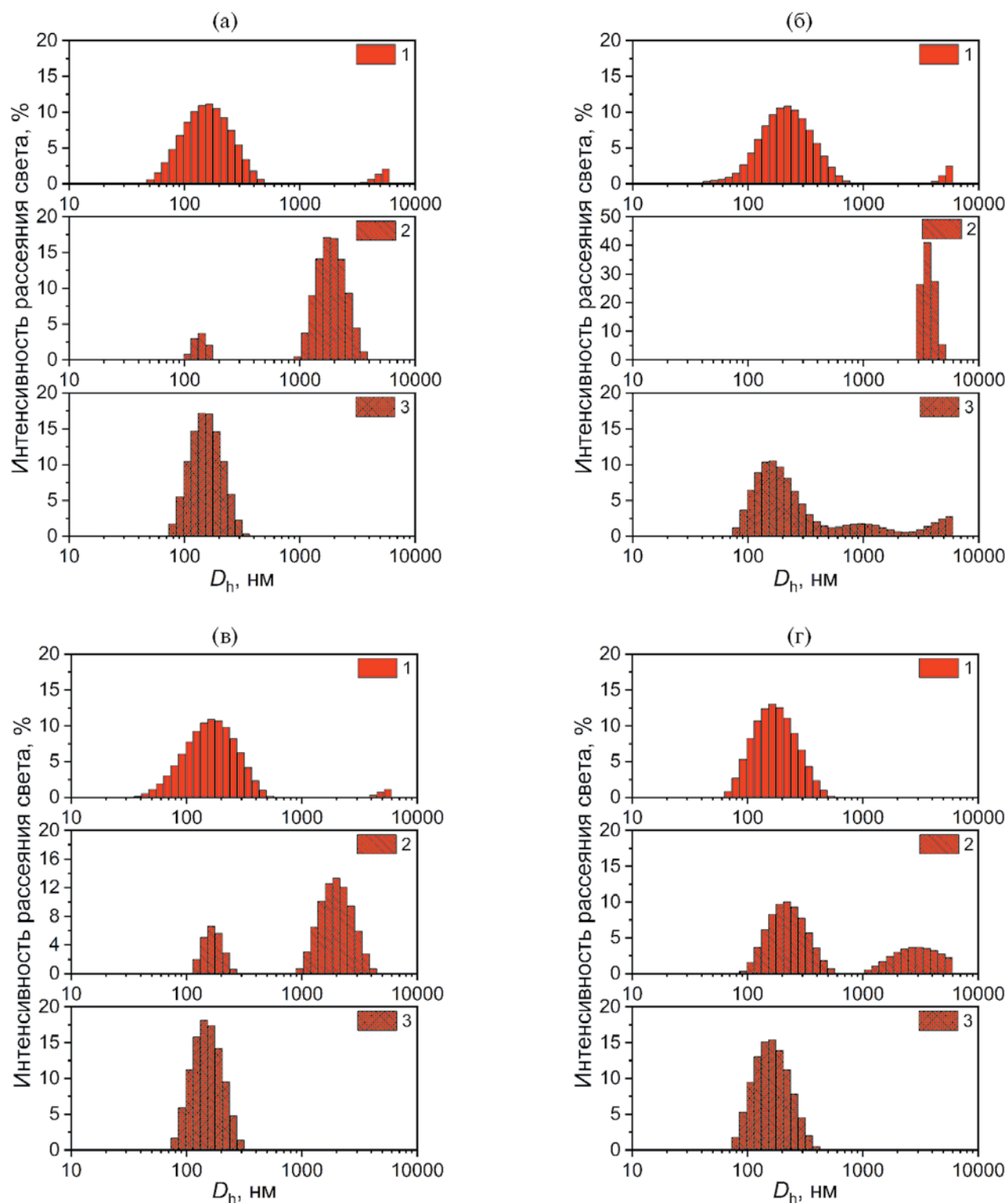
Рис. 4. Распределения интенсивности рассеяния света по гидродинамическим диаметрам ( D_h , нм) ДОЦ-нагруженных ПЛГА-Ві частиц, полученных при концентрации стабилизатора ПВС в водной фазе, равной (а) 1, (б) 5, (в) 10 и (г) 15 мг/мл: 1 – в исходной дисперсии (до лиофилизации), 2 – после лиофилизации без криопротектора и последующего ре-диспергирования в воде, 3 – после лиофилизации в присутствии криопротектора D(–)-маннитола и последующего ре-диспергирования в воде.
