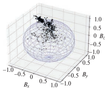
Рис. 2. Графы состояний 15.IV.2023.
