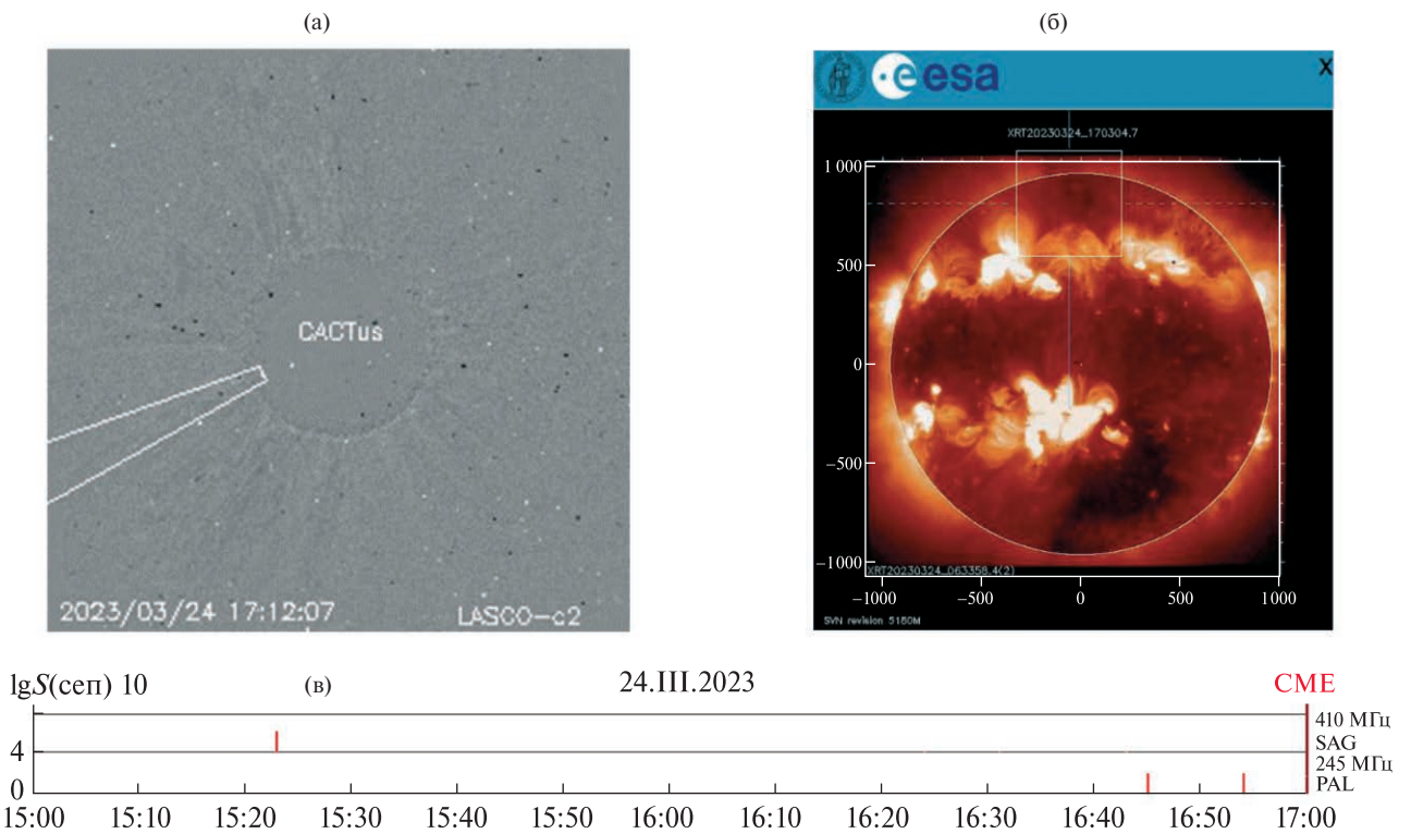
Рис. 8. Пример КВМ, зарегистрированного CACTus (LASCO/C2) 24.III.2023 в 17:00 UT (а), изображение области Солнца в рентгеновских лучах (б) и радиопредвестники КВМ (в).
