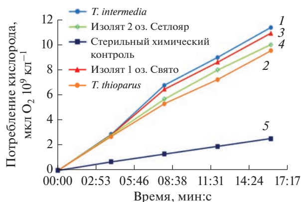
Рис. 4. Окисление сероводорода, измеренное на аппарате Варбурга по потреблению кислорода при 25°C и pH 7 культурами тионовых бактерий Thiomonas intermedia (1) и Thiobacillus thioarous (2) и двух штаммов выделенных из озера гетеротрофных сероокисляющих бактерий (3 – изолят из оз. Свято и 4 – изолят из оз. Светлояр) в сравнении со стерильным химическим окислением (5) (Вайнштейн, 1977). По вертикальной оси: потребление кислорода, мкл O 2 /10 9 кл.; по горизонтальной оси: время, мин.
