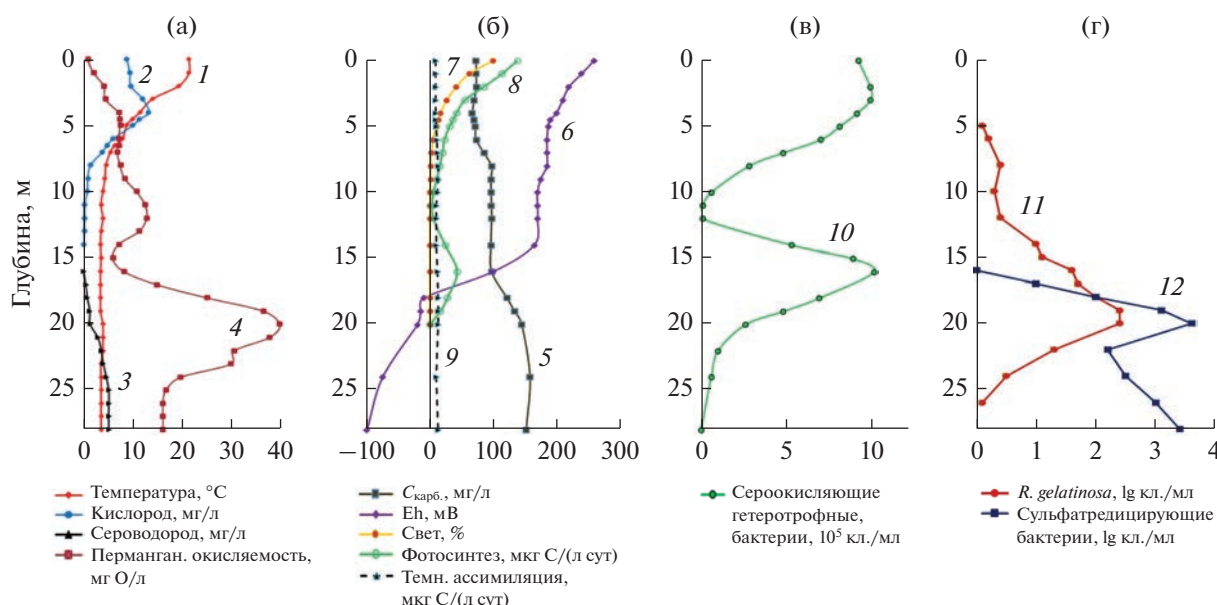
Рис. 3. Гидрохимические характеристики и распределение продукционных процессов и микроорганизмов в водной толще оз. Светлояр. По вертикальной оси – глубина, м. По горизонтальной оси: (а): 1 – температура, °С; 2 – кислород, мг/л; 3 – сероводород, мг/л; 4 – перманганатная окисляемость, мг О 2 /л; (б): 5 – содержание карбонатов, мг/л; 6 – Eh, мВ; 7 – свет, %; 8 – фотосинтез, мкг С/(л сут); 9 – темновая ассимиляция углерода, мкг С/(л сут); (в): 10 – численность сероокисляющих гетеротрофных бактерий, 10 5 кл./мл; (г): численность бактерий: 11 – R. gelatinosa , лг кл./мл; 12 – сульфатредуцирующие бактерии, лг кл./мл.
