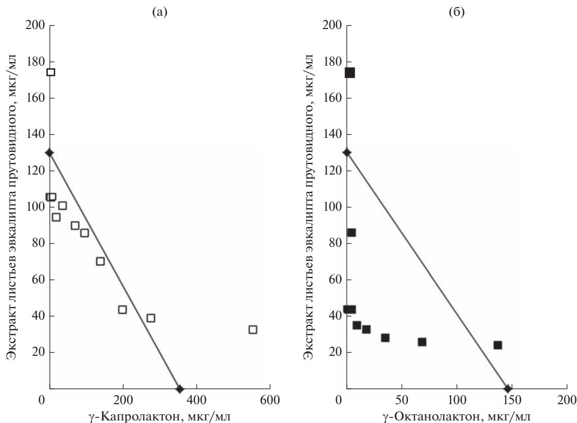
Рис. 3. Изоболографический анализ эффекта комбинаций \gamma -капролактона (а) и \gamma -октанолактона (б) с целым экстрактом листьев эвкалипта прутовидного на QS-контролируемый биосинтез пигмента виолацеина в биотесте на C. subtsugae 026. Изоболы представлены в виде прямых линий, соединяющих значения EC_{50} для каждого отдельного компонента. Результат совместного действия показан путем нанесения на график точек с координатами, соответствующими концентрациям в композиции, обеспечивающим достижение EC_{50} .
