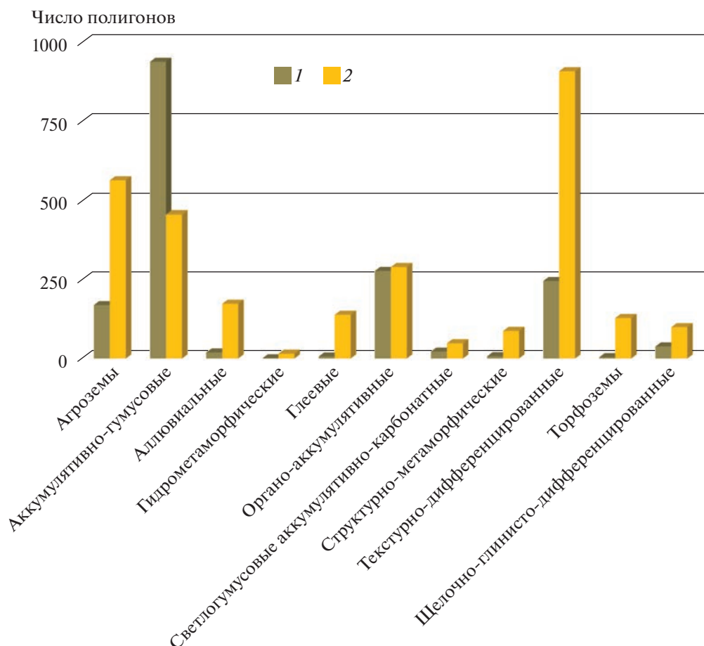
Рис. 3. Количество полигонов с преобладающими (1) и сопутствующими (2) агрогенными почвам разных отделов.
