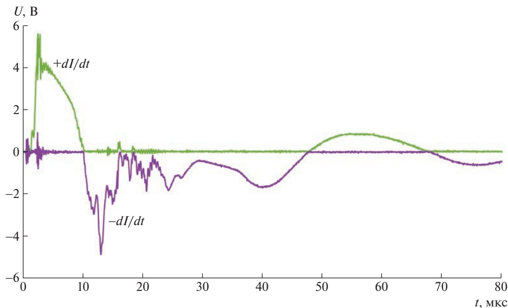
Рис. 5. Сигнал с пояса Роговского.
