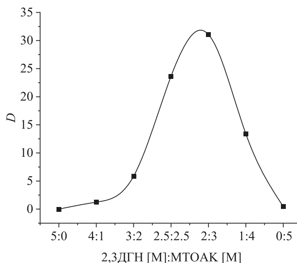
Рис. 2. Зависимость D_Y от соотношения 2,3ДГН и МТОАК. Органическая фаза: 0.005 М изомольярные смеси 2,3ДГН + МТОАК в толуоле, водная фаза: 0.001 М Y_2(CO_3)_3 , 1 М ( Na_2CO_3 + NaOH , pH 12.6).
