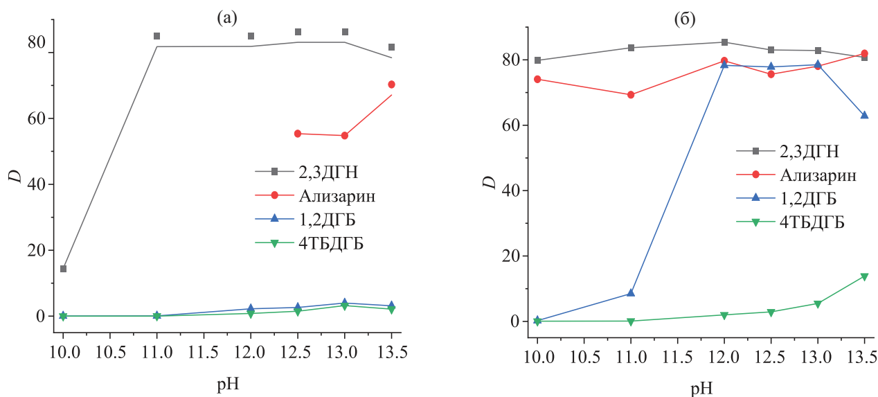
Рис. 3. Зависимость D_Y от pH при экстракции из карбонатных растворов, содержащих 0.001 \text{ M Y}_2(\text{CO}_3)_3 и 1 \text{ M } (\text{Na}_2\text{CO}_3 + \text{NaOH}) смесями, содержащими 0.01 \text{ M} 2,3ДГН, 1,2ДГБ или 4ТБДГБ с 0.015 \text{ M} МТОАК, 0.005 \text{ M} ализарина с 0.01 \text{ M} МТОАК в бутилацетате (а) и толуоле (б).
