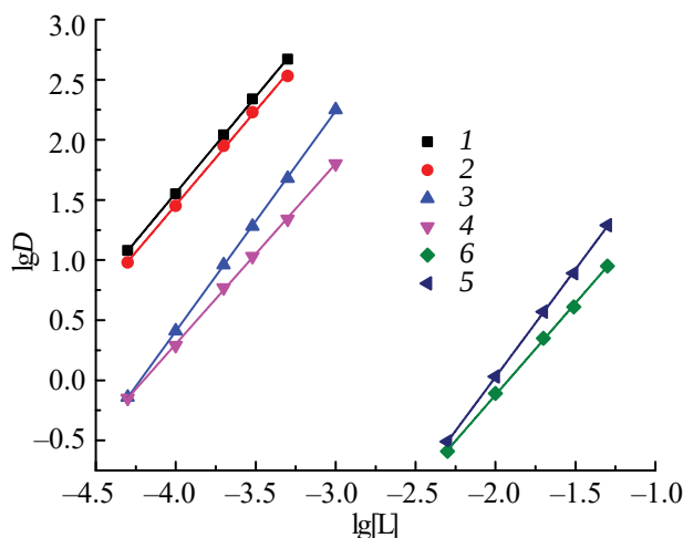
Рис. 2. Зависимость коэффициентов распределения U(VI) (1, 2, 6) и Th(IV) (3–5) от концентрации соединений 2 (1, 3), 4 (2, 4) и 3 (5, 6) в дихлорэтано при экстракции из раствора 3 моль/л \text{HNO}_3 .
