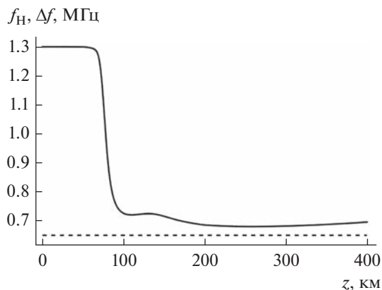
Рис. 17. Зависимости разности частот \Delta f = f_{-} - f_{\text{пл}} (сплошная линия) и полугирочастоты f_{\text{H}}/2 (штриховая) от высоты z .
