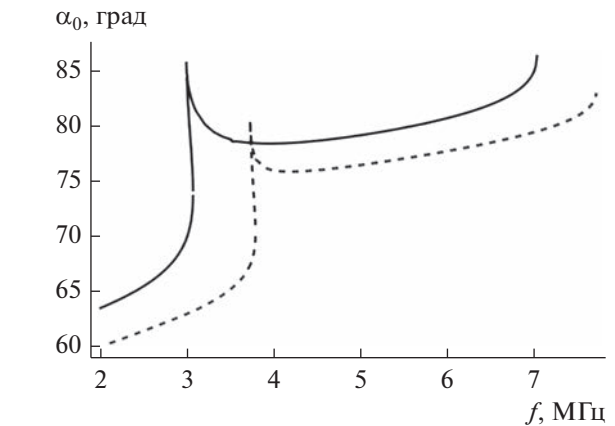
Рис. 7. Зависимость угла выхода сигнала \alpha_0 от частоты f : невозмущенный случай для обыкновенной (сплошная кривая) и необыкновенной волн (штриховая).
