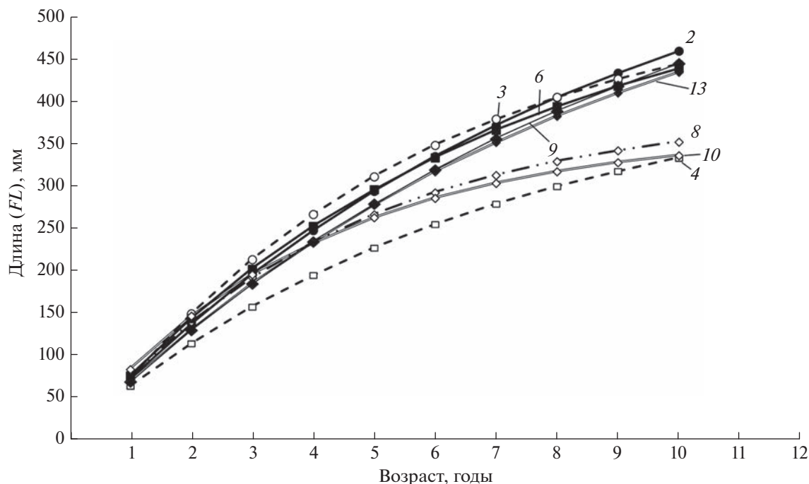
Рис. 3. Кривые линейного роста сига Coregonus lavaretus в разных уральских притоках и озёрах бассейна р. Печора, построенные на основе модели Берталяни.
