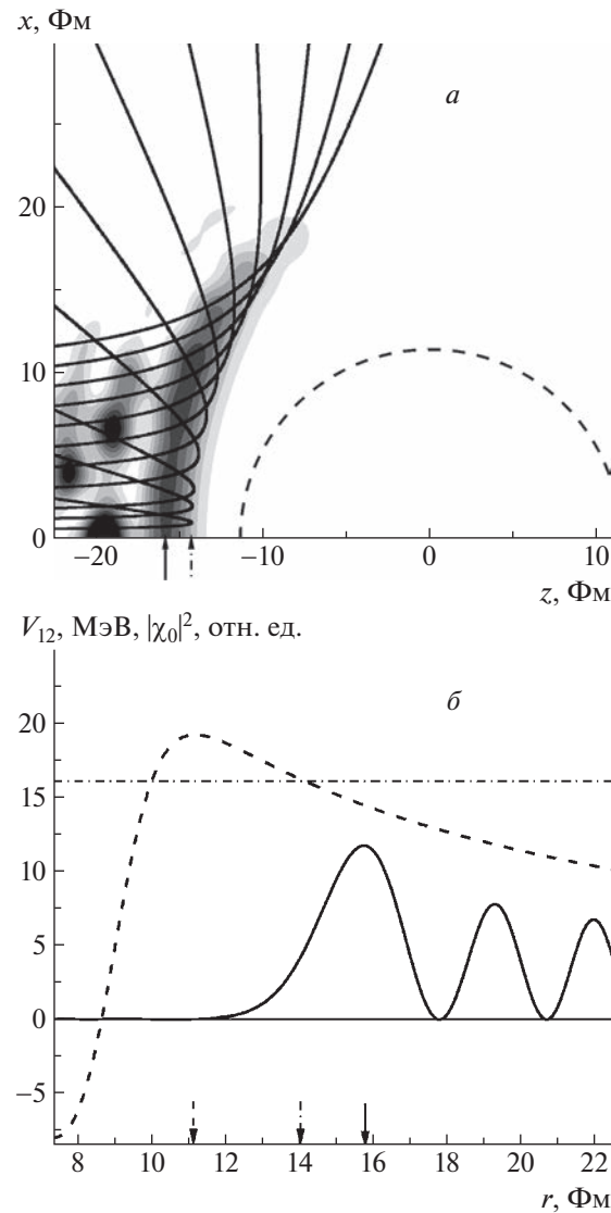
Рис. 1. а — Классические траектории (кривые) и плотность вероятности |\psi_{12}|^2 (оттенки серого) для относительного движения ядер {}^6\text{He} и {}^{197}\text{Au} в ядро-ядерном потенциале V_{12}(r) в системе центра масс при энергии E_{\text{с.м.}} = 16 МэВ, прицельные параметры столкновения 0 < b < 9.5 Фм, орбитальные моменты 0 < l < 20 . Радиус полукруга равен радиусу вершины кулоновского барьера R_B . б — Потенциал V_{12}(r) для системы {}^6\text{He} + {}^{197}\text{Au} (штриховая кривая) и плотность вероятности |\psi_{12}|^2 (сплошная) для орбитального момента l = 0 и E_{\text{с.м.}} = 16 МэВ. Стрелками ( а , б ) отмечены радиус вершины кулоновского барьера R_B , значение R_{\min} при b = 0 (штрихпунктирная) и расстояние R_p пика |\psi_{12}|^2 , ближайшего к центру (сплошная).
