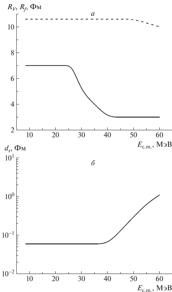
Рис. 5. Зависимости от энергии в системе центра масс E_{c.m.} радиуса R_V области с объемным миним потенциалом для образования ядер ^{198}\text{Au} (сплошная кривая), среднего радиуса R_f слияния ядер (штриховая кривая) (а) и толщины d_s слоя с поверхностным миним потенциалом при R_S = 7.5 Фм для образования ядер ^{196}\text{Au} (б) в реакции ^6\text{He} + ^{197}\text{Au} .
