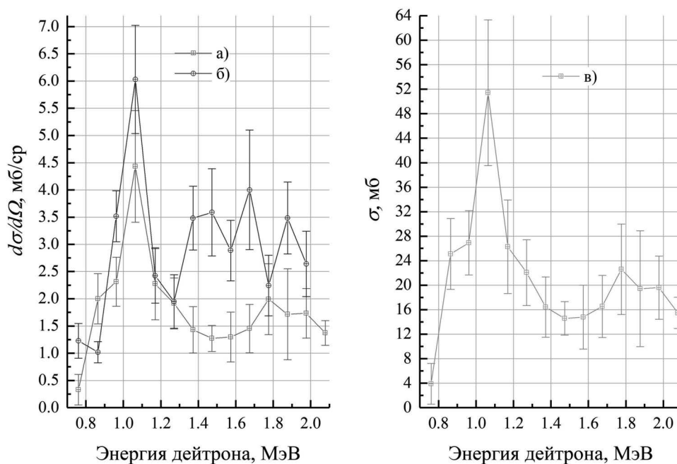
Рис. 6. Дифференциальные (а, б) и эффективное частичное сечения (в) реакции {}^7\text{Li}(d, n){}^8\text{Be}^* с образованием {}^8\text{Be}^* в первом возбужденном состоянии, определенные по измерениям спектров отклика двух алмазных детекторов разной чувствительности с указанием корня суммы квадратов статистической погрешности и погрешности неопределенности функции фона.
