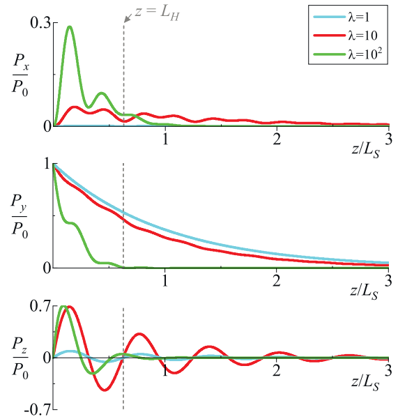
Рис. 4. Поляризация спинового тока в гелимагнетике при \eta = 10 , \lambda = 1; 10; 10^2 , K = +1 для случая инжекции поперечно-поляризованного спинового тока с поляризацией на границе P_x = P_z = 0 , P_y = P_0
