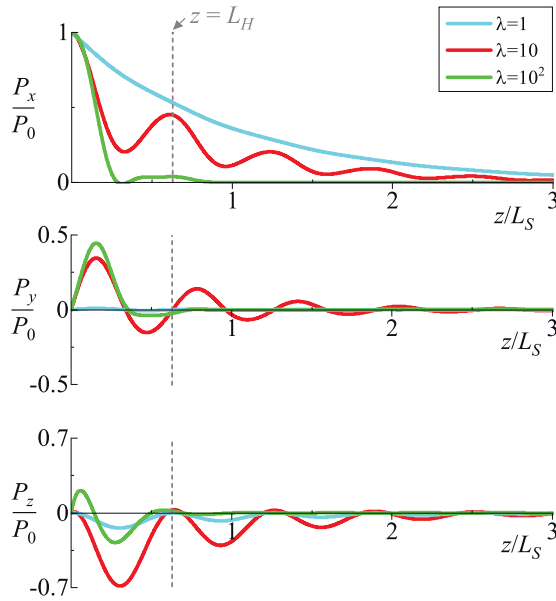
Рис. 3. Поляризация спинового тока в гелимагнетике при \eta = 10 , \lambda = 1; 10; 10^2 , K = +1 для случая инжекции спинового тока, имеющего поляризацию \mathbf{P}_0 = P_0 \mathbf{h}_0
