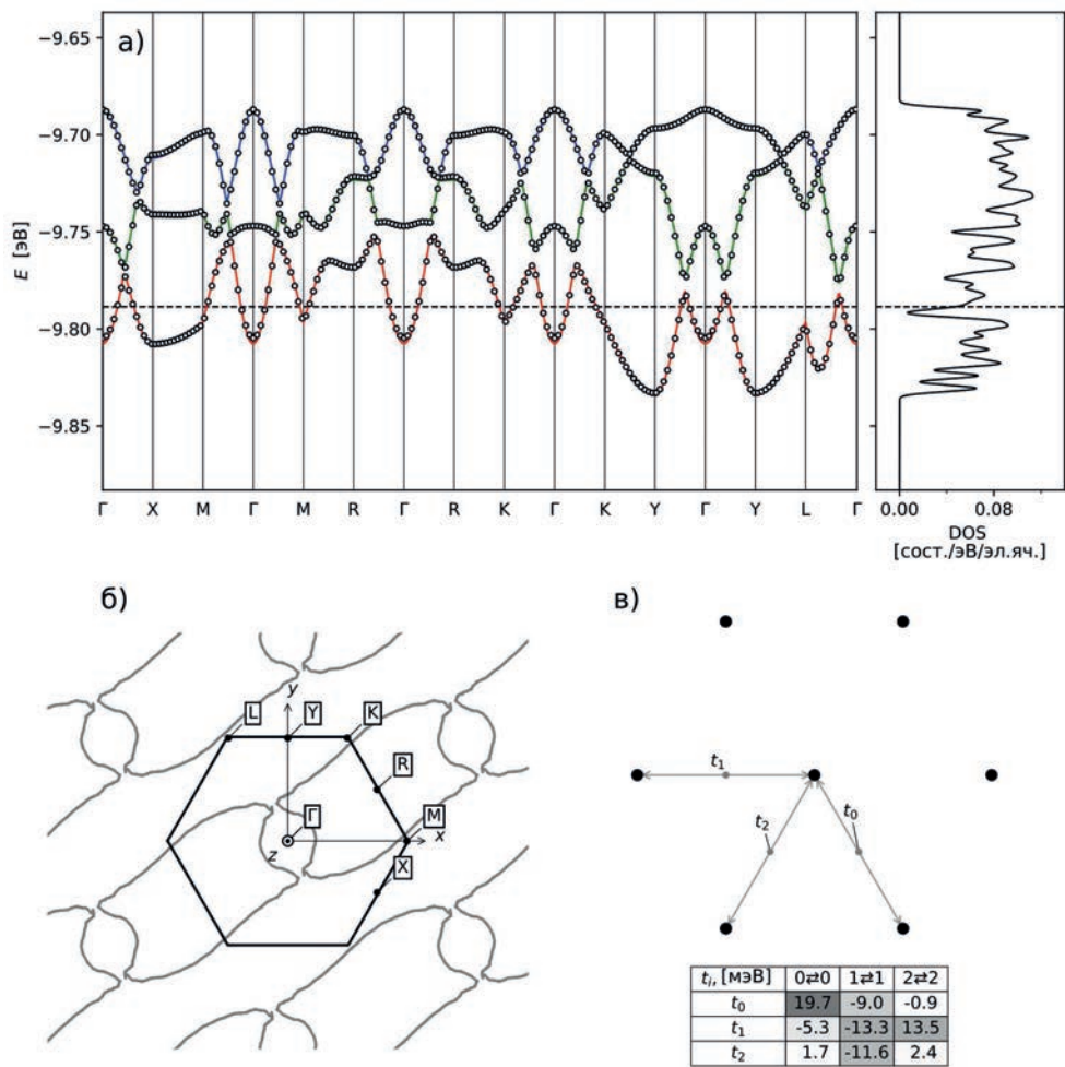
Рис. 3. Зонная структура, плотность состояний (а), поверхность Ферми (б) и интегралы переноса t_i (в) для слоя В кристалла C_{60}^{\bullet-} -MDABCO ^{+} -TPC-I
