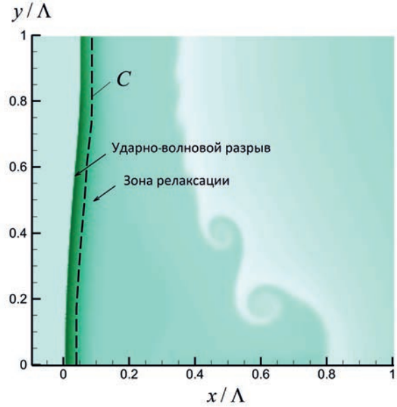
Рис. 4. Положение контура C , на котором вычисляют среднеквадратичные пульсации давления за фронтом ударной волны
