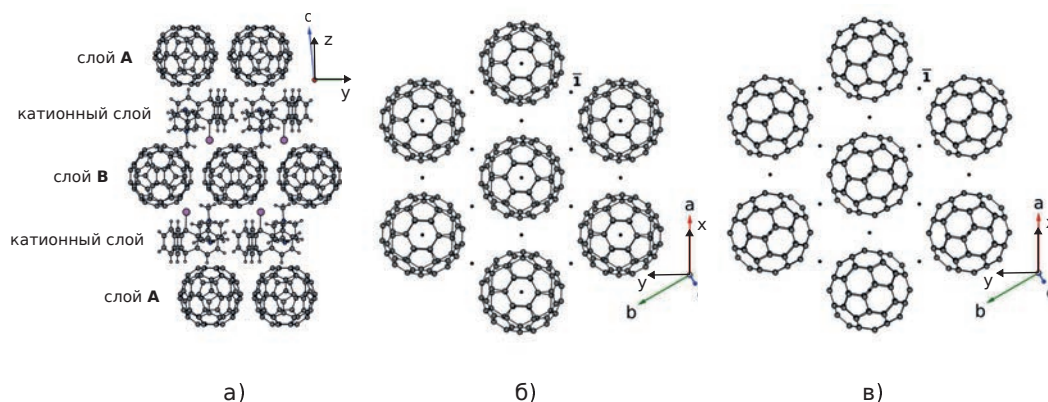
Рис. 1. a — Слоистая структура кристаллов C_{60}^{\bullet-} -MDABCO + -TPC-I; b — вид слоя А вдоль направления c^* ; c — вид слоя В вдоль направления c^* ; a , b , c — направления кристаллографических осей координат, x , y , z — декартова система координат, соответствующая кристаллографической
