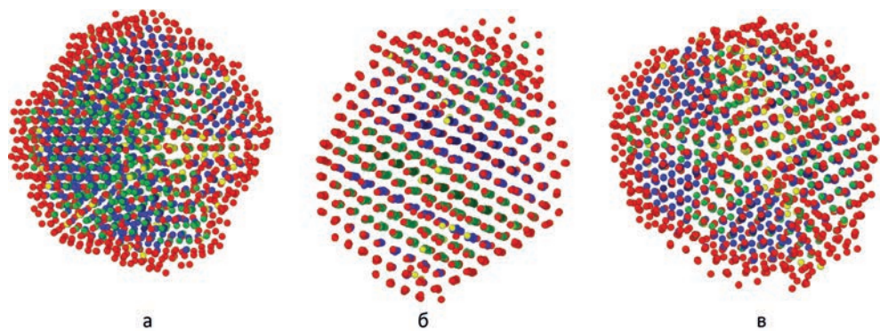
Рис. 2. (В цвете онлайн) Примеры кристаллических структур нанокластеров Ag 50 Au 50 диаметром 4.0 нм, полученные в ходе охлаждения из расплава: Ih (а), ГЦК/ГПУ (б), Dh (в). Разный цвет атомов серебра определяется стандартной СНА-методикой, анализирующей число связей каждого атома в первой, второй и третьей координационных сферах. Так, атом красного цвета обозначает, что его координационное число в первой сфере меньше 12, атом желтого цвета — что его координационное число в первой сфере равно 12, но во второй меньше значения, характерного для плотноупакованных структур (ГЦК, ГПУ). Атомы синего цвета показывают, что их координационные числа в первой, второй и третьей координационных сферах соответствуют ГЦК-структуре, а зеленого — ГПУ
