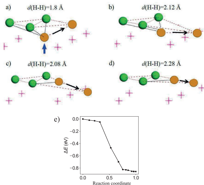
Рис. 8. a, b, c, d — Рост малого кластера за счет выхода атома H из массива (на рис. 8 a показан синей стрелкой). Черной стрелкой показано направление выталкивания одного из атомов кластера на его периферию; e — изменение энергии системы в процессе перемещений, представленных на рис. 8 a, b, c, d (за уровень отсчета принята энергия начальной конфигурации системы, соответствующая рис. 8 a )
