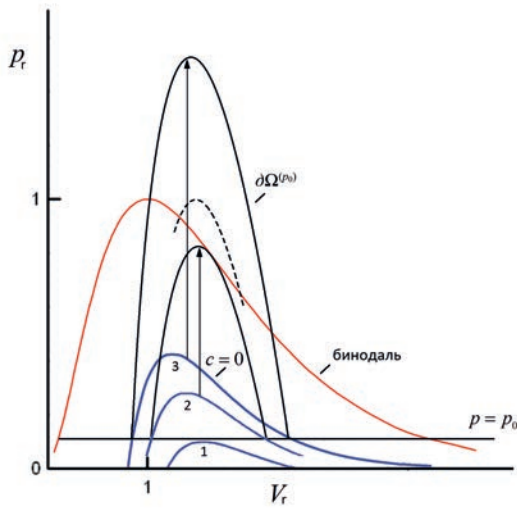
Рис. 3. Схема, показывающая зависимость области нейтральной устойчивости \partial\Omega^{(p_0)} в реальных газах от изохорной теплоемкости. Кривые 1–3 — адиабатическая спинодаль для трех значений теплоемкости c_{V3} > c_{V2} > c_{V1} . \Omega^{(p_0)} для каждого значения c_V определяется неравенством (43)
