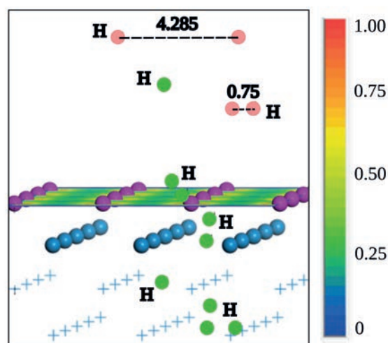
Рис. 1. Различные начальные положениями одного атома H (зеленые шарики) и пар атомов H (розовые шарики) с разным межатомным расстоянием относительно поверхности W(100). Представлена цветовая карта распределения электронной плотности на поверхности в интервале [0-1] электрон/ \text{\AA}^3 . Атомы W верхнего слоя поверхности здесь и далее изображены фиолетовыми шариками, атомы W второго слоя и более глубоких слоев под поверхностью изображаются синими крестиками (либо синими шариками)
