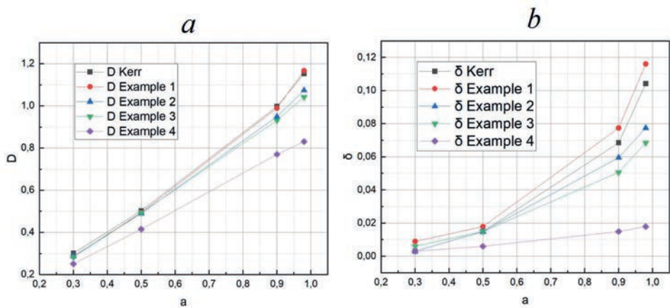
Рис. 3. Зависимости смещения D (a) и параметра искажения \delta (b) от параметра вращения a для случая метрики Керра и различных фиксированных полей при угле наклона плоскости вращения \theta_0 = \pi/2
