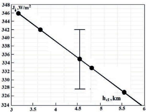
Рис. 1. Зависимость потока излучения из атмосферы на поверхность Земли J_\downarrow от высоты границы облаков h_{cl} . Кружки соответствуют пяти источникам энергетического баланса Земли и ее атмосферы
