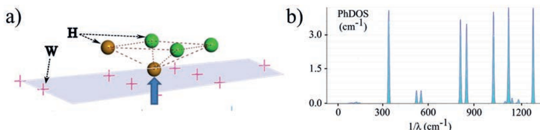
Рис. 7. a — Кластер из четырех адсорбированных атомов H и «всплывший» из массива под кластер атом водорода (выделен жирной стрелкой); b — парциальный спектр колебаний системы из атомов водорода, представленной на рис. 7 a . Рекомбинирующая пара атомов H (здесь и на рис. 8) выделена коричневым цветом
