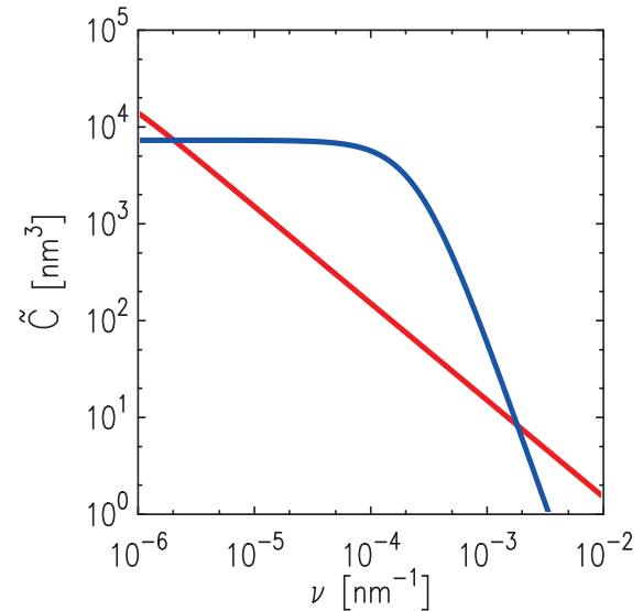
Рис. 6. Компоненты спектров корреляционной функции шероховатости \tilde{C}(\nu) для капиллярно-волновой структуры на межфазной границе (красная линия) и для мицеллярного слоя (синяя линия)
