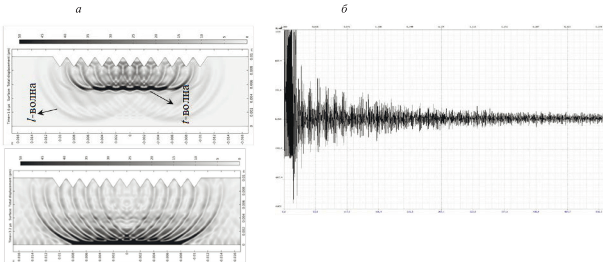
Рис.1. Результат моделирования акустического поля в плоскости поперечного сечения образца с резьбой в различные моменты времени (0,18 мкс и 0,71 мкс) (а), осциллограмма при контроле резьбы (б).
