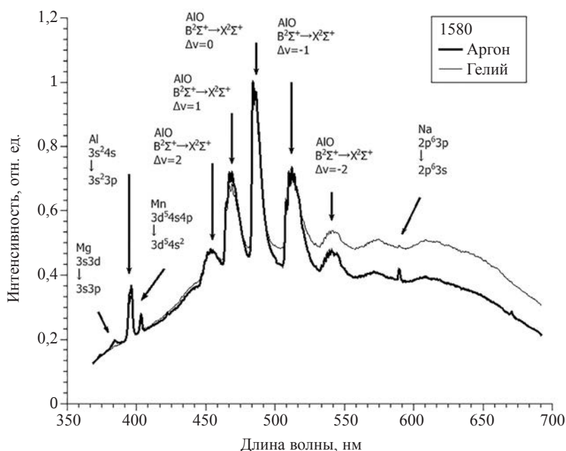
Рис. 3. Нормированные на максимум спектры, измеренные при лазерном воздействии на образцы сплава 1580 при использовании гелия или аргона в качестве защитного технологического газа.
