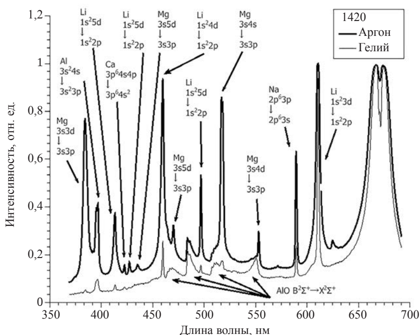
Рис. 2. Нормированные на максимум спектры, измеренные при лазерном воздействии на образцы сплава 1420 при использовании гелия или аргона в качестве защитного технологического газа.
