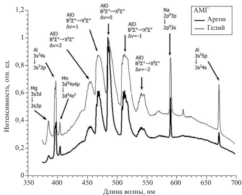
Рис. 4. Нормированные на максимум спектры, измеренные при лазерном воздействии на образцы сплава АМг6 при использовании гелия или аргона в качестве защитного технологического газа.
