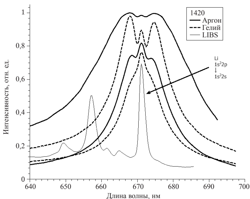
Рис. 5. Фрагмент спектра сплава 1420 для двух различных измерений при воздействии непрерывным излучением волоконного лазера с различными технологическими газами и искровом пробое (LIBS), вызванном импульсным излучением углекислотного лазера.
