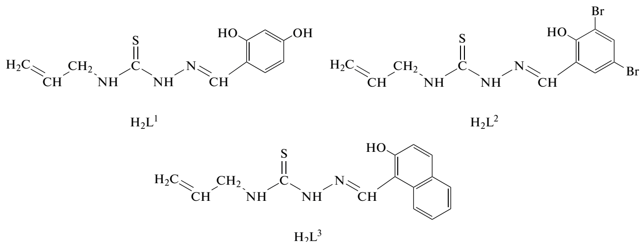
Рис. 3. Строение 4-аллилтиосемикарбазонов 2,4-дигидроксibenзальдегида ( H_2L^1 ), 3,5-дибромсалицилового альдегида ( H_2L^2 ) и 2-гидрокси-1-нафталъдегида ( H_2L^3 ) [25].
