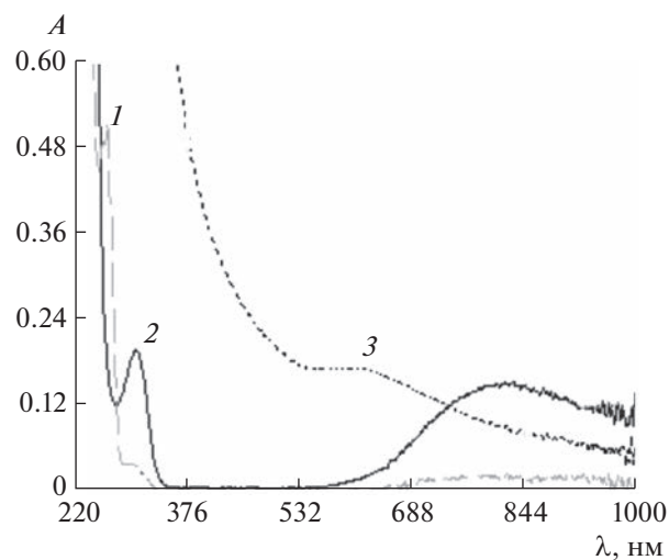
Рис. 2. Зависимость оптической плотности ( A ) от длины волны ( \lambda ) олигомера (лиганда) с медью в водной среде: 1 – олигомер на основе морфолина с эпихлоргидрином, 2 – нитрат меди, 3 – смесь олигомера с нитратом меди(II) [23].
