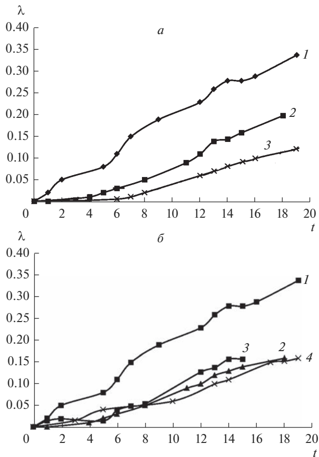
Рис. 4. Изменение относительного расширения \lambda (%) с течением времени t (сут) для цементно-песчаных растворных смесей на основе песка 2, содержащего метакраин (а) и микрокремнезем (б), в необработанном состоянии (1) и подвергнутого ЭЛО при значениях поглощенной дозы 100 (2), 300 (3) и 600 кГр (4).
