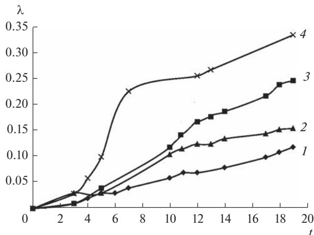
Рис. 1. Изменение относительного расширения \lambda (%) с течением времени t (сут) для цементно-песчаных растворов на основе песка 1 в необработанном состоянии (1) и подвергнутого ЭЛО при значениях поглощенной дозы 100 (2), 300 (3) и 600 кГр (4).
