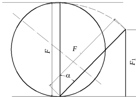
Рис. 1. Схема расчета удельной площади воздействия на пузырек: F – условный размер лопасти; F_1 – эффективный условный размер лопасти; \alpha – угол наклона лопасти, град.
