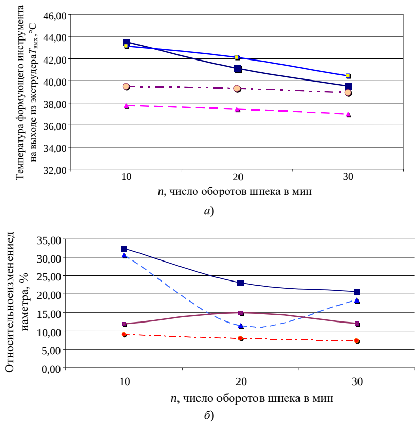
Рис. 3. Зависимости температуры формующего инструмента на выходе из формующей головки T_{\text{вых}} (а) и относительного изменения диаметра \delta до и после его охлаждения (б) от частоты вращения шнека n :
