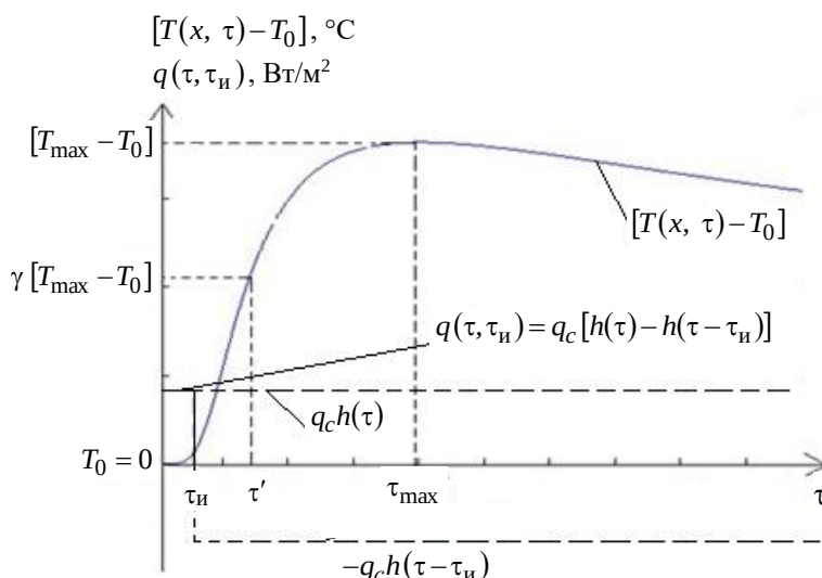
Рис. 1. Изменение во времени \tau физических величин: теплового импульса q(\tau, \tau_n) = q_c [h(\tau) - h(\tau - \tau_n)] , представляющего собой алгебраическую сумму ступенчатых функций q_c h(\tau) и -q_c h(\tau - \tau_n) ; разности температур [T(x, \tau) - T_0] на расстоянии x от плоского импульсного источника теплоты
