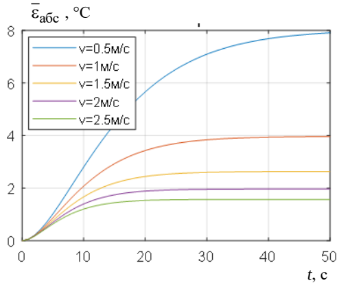
Рис. 5. Влияние скорости воздуха на изменение абсолютной погрешности расчета температуры спирали при ее нагреве
