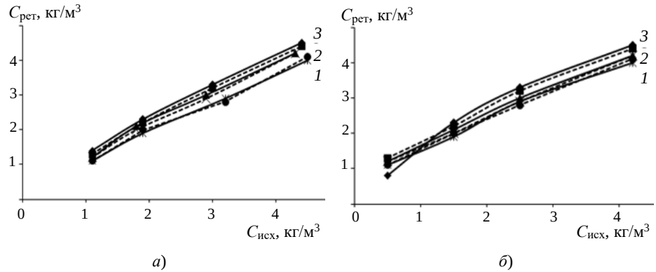
Рис. 4. Сопоставление экспериментальных и расчетных данных концентрационных зависимостей от давления для мембраны МФФК-0 при температуре T = 293 К для раствора тринатрийфосфата (а) и триполифосфата (б) P , МПа: 1 – 0,1; 2 – 0,15; 3 – 0,20 (сплошные линии – эксперимент, штриховые – расчет)
