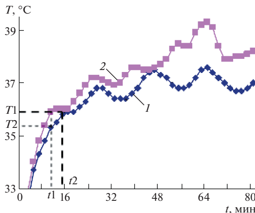
Рис. 2. График зависимости температуры в области тканого электронагревателя, находящегося на поверхности тела человека, от времени, полученной экспериментальным путем при различных уровнях воздействующего сигнала: 1 – при максимальном уровне меньше 38^\circ\text{C} ; 2 – при максимальном уровне больше 38^\circ\text{C} .
