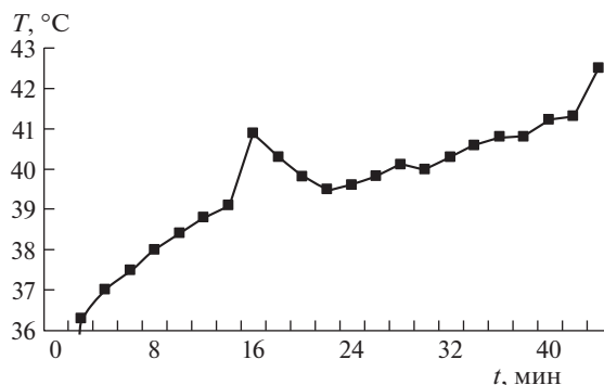
Рис. 5. Изменение температуры на поверхности тела человека при подаче теплового сигнала более мощного, чем вызывающего только потовыделение.
