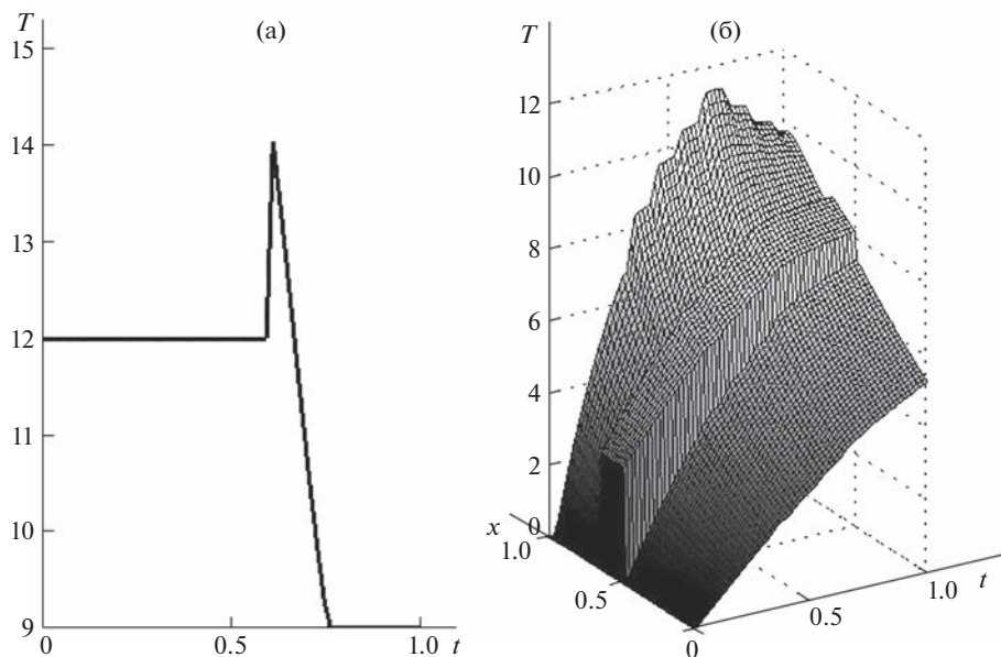
Рис. 4. График изменения температуры во времени, полученный с помощью тепловой модели на поверхности нагревателя при более высоком уровне теплового воздействия, более 38^{\circ}\text{C} : (а) — модель воздействующего со стороны человека теплового сигнала; (б) — характер изменения теплового поля во времени и по пространству тонкой стенки.
