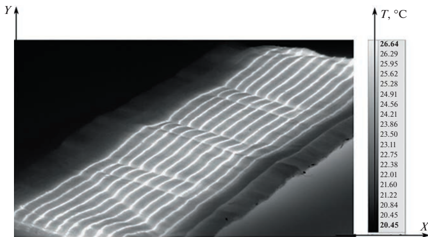
Рис. 1. Изменение температуры на поверхности тканого электронагревателя.
