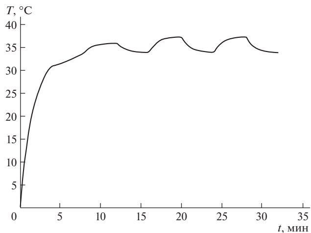
Рис. 3. График изменения температуры, полученный с помощью тепловой модели на поверхности нагревателя при небольшом уровне теплового воздействия.
