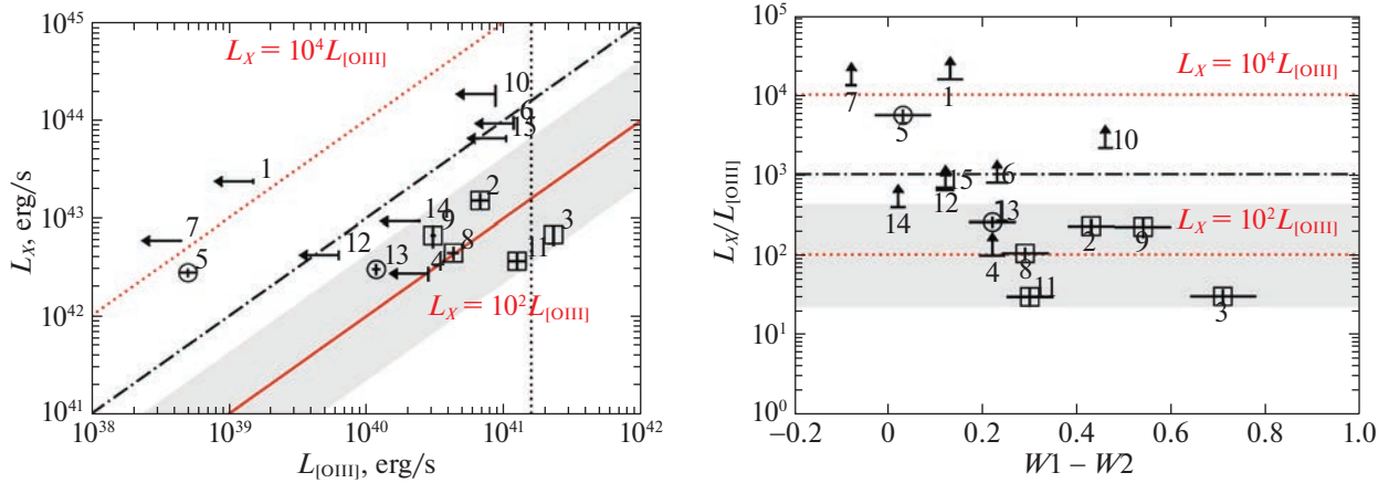
Рис. 3. Слева: Рентгеновская светимость, L_X , рассчитанная через значение максимального потока в обзоре СРГ/еРОЗИТА, и светимость в линии [ОIII] (5007 Å), L_{\text{[OIII]}} . Справа: Отношение L_X/L_{\text{[OIII]}} в зависимости от ИК цвета W1-W2 (Vega). Кружками отмечены объекты, в спектре которых есть только узкие эмиссионные линии, квадратами — объекты, в спектре которых есть хотя бы одна широкая бальмеровская линия. Для объектов, в спектре которых отсутствует линия [ОIII] (5007 Å), показаны соответствующие верхние пределы. Вертикальной линией \lg(L_{\text{[OIII]}}/A.2) показана эмпирическая граница между АЯГ и звездообразующими галактиками для обзора GAMA (Яо и др., 2020). Серым цветом закрашена область, в которой обычно располагаются АЯГ: в среднем \lg(L_{\text{[OIII]}}/L_X) = -1.99 , с разбросом \sigma = 0.63 (Яо и др., 2015), а черным штрихпунктиром — отношение L_X/L_{\text{[OIII]}} = 10^3 , которое мы предлагаем использовать для отделения кандидатов в СПР (более высокие значения) от АЯГ.
