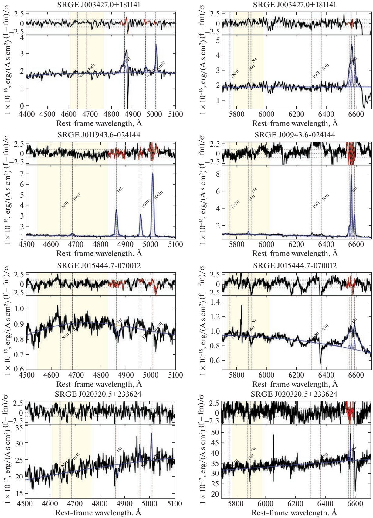
Рис. 5. Подгонка параметров моделей спектральных линий.
