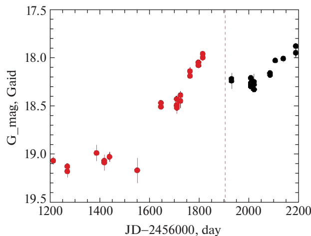
Рис. 2. Оптическая кривая блеска SGR J143701.5+264019 (квазар). Красными кружочками показаны данные, соответствующие периоду каталога Gaia eDR3.
