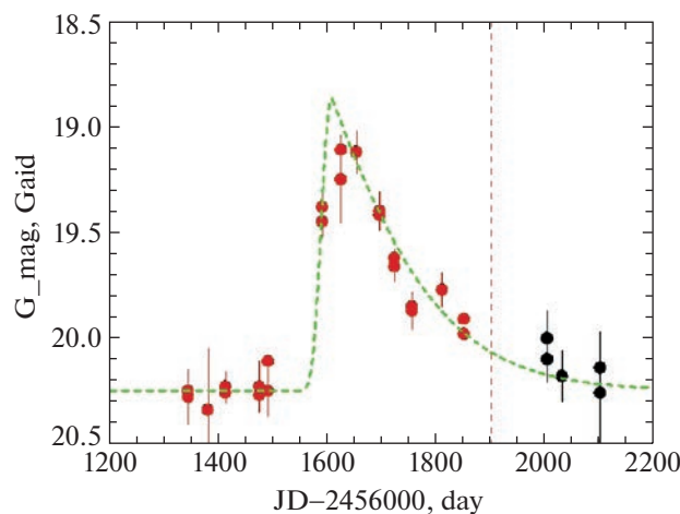
Рис. 3. Оптическая кривая блеска SGR J151721.7+465812 (галактика со звездообразованием). Красными кружочками показаны данные, соответствующие периоду каталога Gaia eDR3. Зеленым пунктиром — подгонка вспышки с FRED-профилем.
