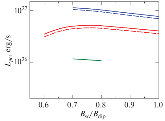
Рис. 5. То же, что на рис. 2, но при W_0 = 6 \times 10^5 \text{ c}^{-1} и f = 0.1 .
