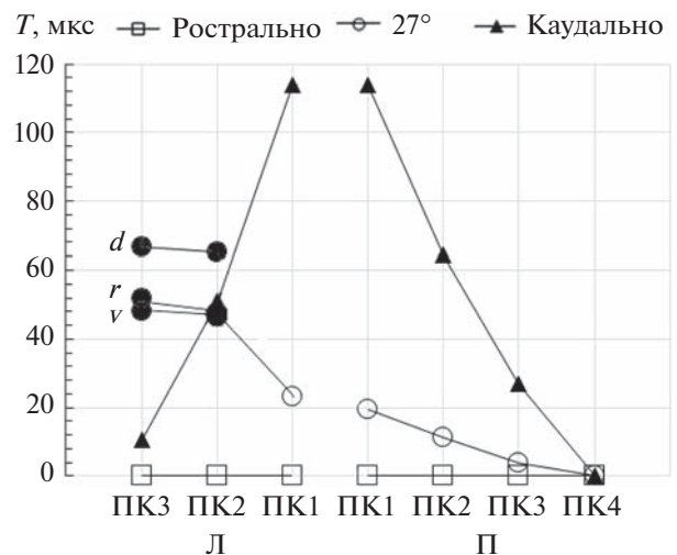
Рис. 3. Относительное время задержки парциальных звуков ПК1–ПК3 левого (Л) и ПК1–ПК4 правого (П) наружного уха, для роstralного, каудального, и под углом 27^\circ к оси X звука во фронтальной плоскости (рис. 1), соответственно. Ось ординат — время задержки T в мкс. Ось абсцисс — номера соответствующих ПК. Маркеры, не залитые (залитые) черным, означают освещение звуком (экранирование роstrумом) соответствующих ПК. Обозначения d , r и v указаны на рис. 2.
