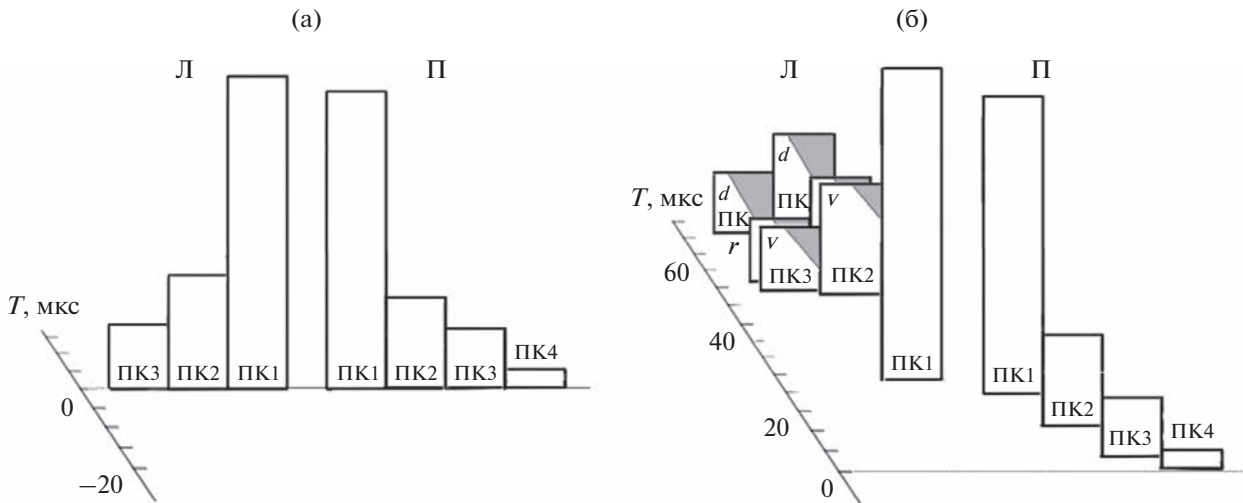
Рис. 2. Относительное время задержки парциальных звуков ПК1–ПК3 левого (Л) и ПК1–ПК4 правого (П) наружного уха, (а) — для роstralного и (б) — под углом 27^\circ к оси X звука во фронтальной плоскости (рис. 1а), соответственно. Высота прямоугольников пропорциональна уровням относительных звуковых давлений парциальных звуков, ширина прямоугольников эквивалентна полосе частот слуха дельфина (1–160 кГц). Результаты спектральной фильтрации парциальных звуков закрашены. Длительность звука в ПК одинакова, условно не показана. T — время задержки в мкс. d , r и v — дифракция звука с дорсальной, вентральной и роstralной стороны наружных ушей (роstrума) на контралатеральные ПК, соответственно.
