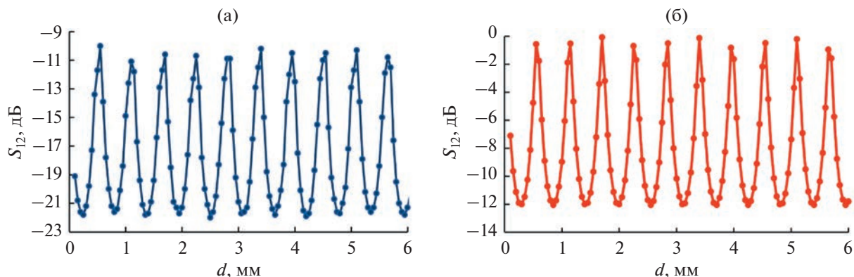
Рис. 2. (а) — Экспериментальная и (б) — теоретическая зависимости параметра S_{12} от расстояния d между пьезопреобразователями для этилового спирта.
