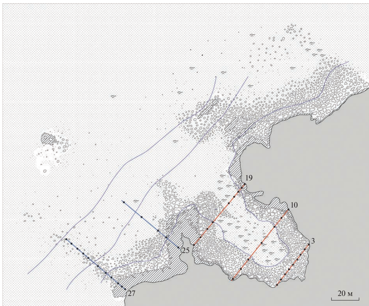
Рис. 2. Схема рельефа и грунтов залива Крестового и расположение разрезов. Разрезы 3, 10 и 19 проходят через мелководную полужакрытую бухту. Разрезы 25 и 27 расположены на свале открытого побережья. Остальные обозначения, как на рис. 1.
