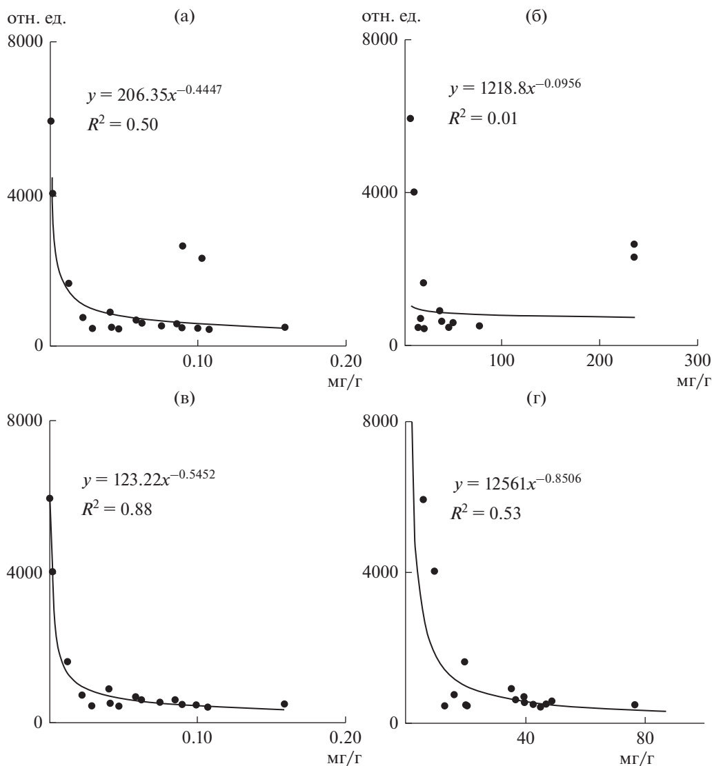
Рис. 3. Связи C/(Xл + \Phi) с содержанием пигментов и органического углерода в Увдовском водохранилище. По оси ординат – отношение C/(Xл + \Phi) ; по оси абсцисс: а – Xл + \Phi , мг/г с.о., для всех проб, б – ОВ , мг/г с.о., для всех проб, в – Xл + \Phi , мг/г с.о., без торфянистого ила, г – ОВ , мг/г с.о., без торфянистого ила.
