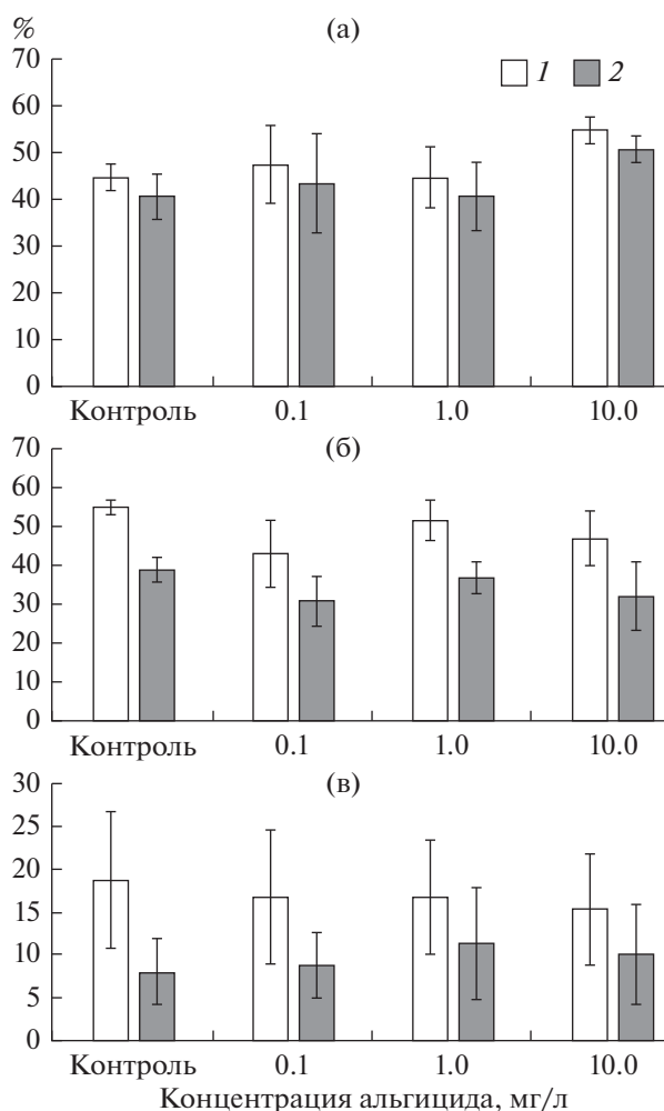
Рис. 1. Изменение важнейших показателей прорастания (ось y) — конечного прорастания ( G_{fin} ) и энергии прорастания (E, %) при действии различных концентраций альгицида на семена Sparganium emersum (а), S. glomeratum (б) и Schoenoplectus lacustris (в). 1 — G_{fin} , 2 — E.
