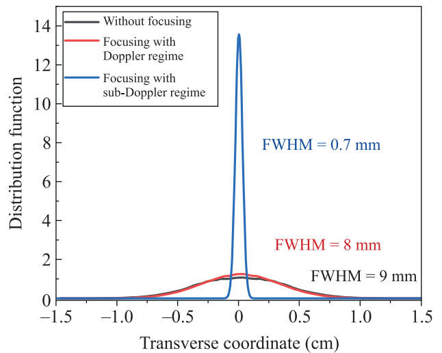
Рис. 3. (Цветной онлайн) Функция пространственного распределения плотности атомов вдоль поперечной оси X в фокальной плоскости: (1) без фокусировки (черная кривая); (2) фокусировка в 2D-МОЛ при доплеровском режиме охлаждения (красная кривая); (3) фокусировка в 2D-МОЛ при суб-доплеровском механизме охлаждения (синяя кривая)
