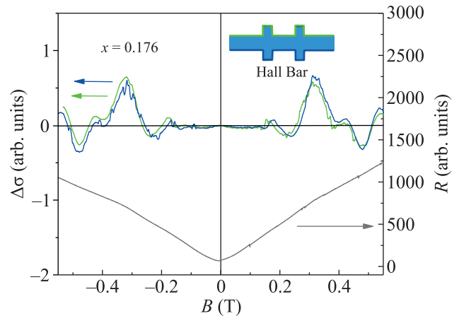
Рис. 2. (Цветной онлайн) Зависимость фотопроводимости образца с составом x = 0.175 от магнитного поля для различных пар потенциальных контактов на образце (зеленая и синяя кривые, левая ось); магнитолевая зависимость сопротивления образца в равновесных условиях (серая кривая, правая ось)
