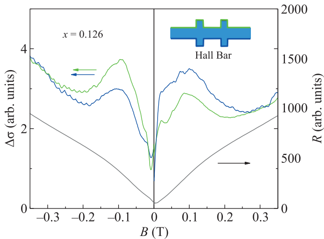
Рис. 1. (Цветной онлайн) Зависимость фотопроводимости образца с составом x = 0.126 от магнитного поля для различных пар потенциальных контактов на образце (зеленая и синяя кривые, левая ось); магнитолевая зависимость сопротивления образца в равновесных условиях (серая кривая, правая ось)
