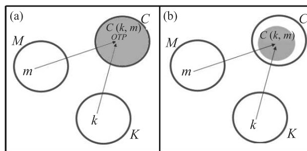
Рис. 1. (Цветной онлайн) Схематическое изображение множеств (инвариантов) шифр-текстов для: (а) – любой реализации шифрования одноразовым блокнотом C_{OTP}(k, m) (OTR сокращение от One Time Pad); (б) – блочным шифром c(k, m)
