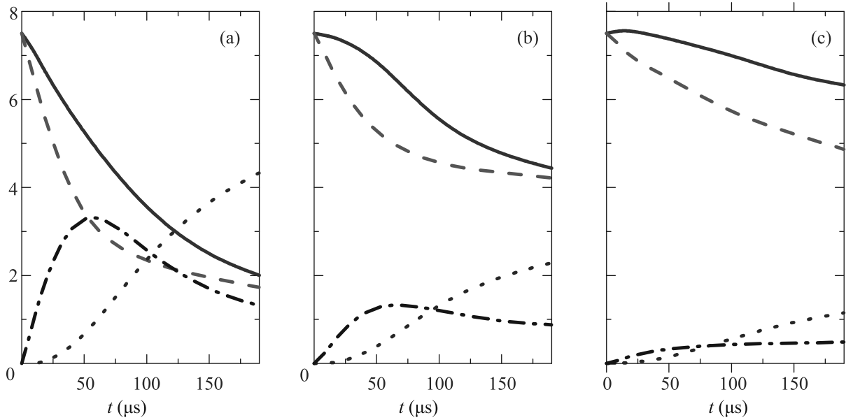
Рис. 3. (Цветной онлайн) Средние значения (в градусах Кельвина) на одну частицу кинетической энергии электронов и ионов плазмы E_{\text{kep}} (синие сплошные), E_{\text{kip}} (коричневые точечные), кинетической энергии улетевших электронов E_{\text{kout}} (красный пунктир) и полной потенциальной энергии U : (a) – B = 0 Гс/см; (b) – B = 30 Гс/см и (c) – B = 500 Гс/см. T_{e0} = 5 К
