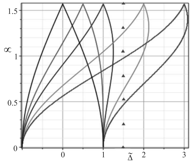
Рис. 1. (Цветной онлайн) Фазовая диаграмма пленки АФМ ТИ в зависимости от параметров модели. Вдоль вертикальной оси отложен угол неколлинеарности \alpha , вдоль горизонтальной – безразмерная энергия гибридизации \tilde{\Delta} = \frac{\Delta_0}{M_\perp m_0} . Кривые линии ограничивают область КАЭХ. Справа от области КАЭХ располагается область КСЭХ, слева – область тривиального изолятора. Безразмерный параметр \gamma = \frac{M_\parallel^2}{M_\perp^2} \frac{bM_\perp m_0}{\mathcal{A}^2} принимает значения: 0 (черная кривая), 0.5 (красная), 1 (синяя), 2 (зеленая), 3 (коричневая)
