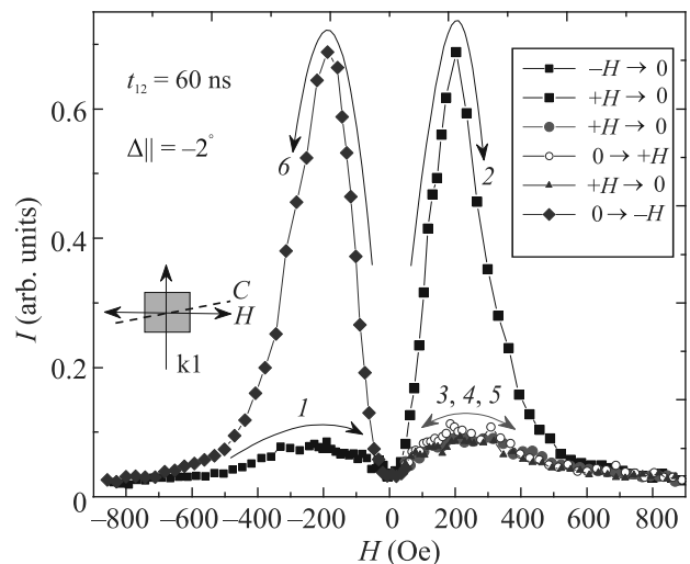
Рис. 1. (Цветной онлайн) Интенсивность ФЭ в \text{LuLiF}_4:\text{Er}^{3+} ( 0.025\text{ ат. \%} ) для импульсов \pi -поляризации. Угол \angle(C, H) = -2^\circ . Видно, что I(H \downarrow) = I(H \uparrow) (кривые 3, 4, 5) при повторных измерениях в поле одной полярности, а при смене полярности магнитного поля происходит однократное (зеркальное относительно оси H = 0 ) изменение I(H \uparrow) (кривые 2 и 6)
