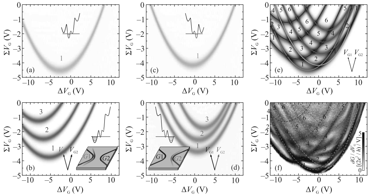
Рис. 3. (Цветной онлайн) (a)–(d) – Транскондактанс \partial G/\partial(\Sigma V_G) четырех отдельных параллельных проводящих каналов, как функция разности \Delta V_G и суммы \Sigma V_G затворных напряжений. (e) – Суммарный транскондактанс четырех каналов. (f) – Экспериментально измеренный транскондактанс. Штриховые линии соответствуют линиям, показанным на (e). Светлые области соответствуют плато. Целые числа на графиках показывают значения кондактанса в единицах 2e^2/h . Вставки показывают соответствующие минимумы в четырехъямном ограничивающем потенциале и положение соответствующего канала внутри КТК
