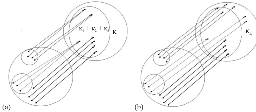
Рис. 1. (Цветной онлайн) (а) – Схематическое изображение множества ключей и шифр-текстов для блочного шифра; (б) – схематическое изображение множества ключей и шифр-текстов для одноразового блокнота
